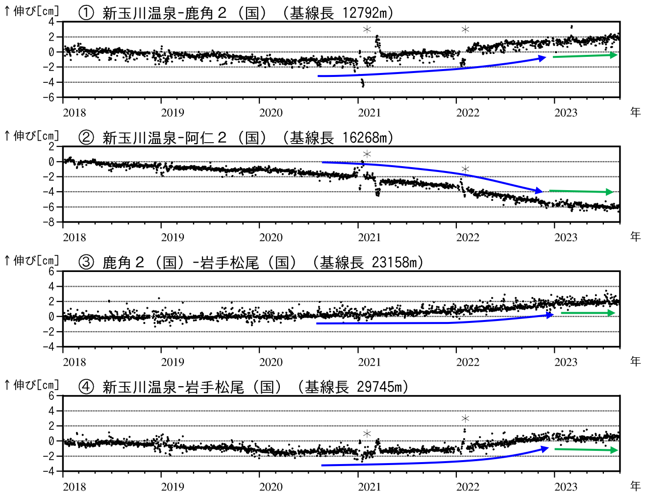
図4 秋田焼山 GNSS 基線長変化図（2018年1月～2023年8月）
