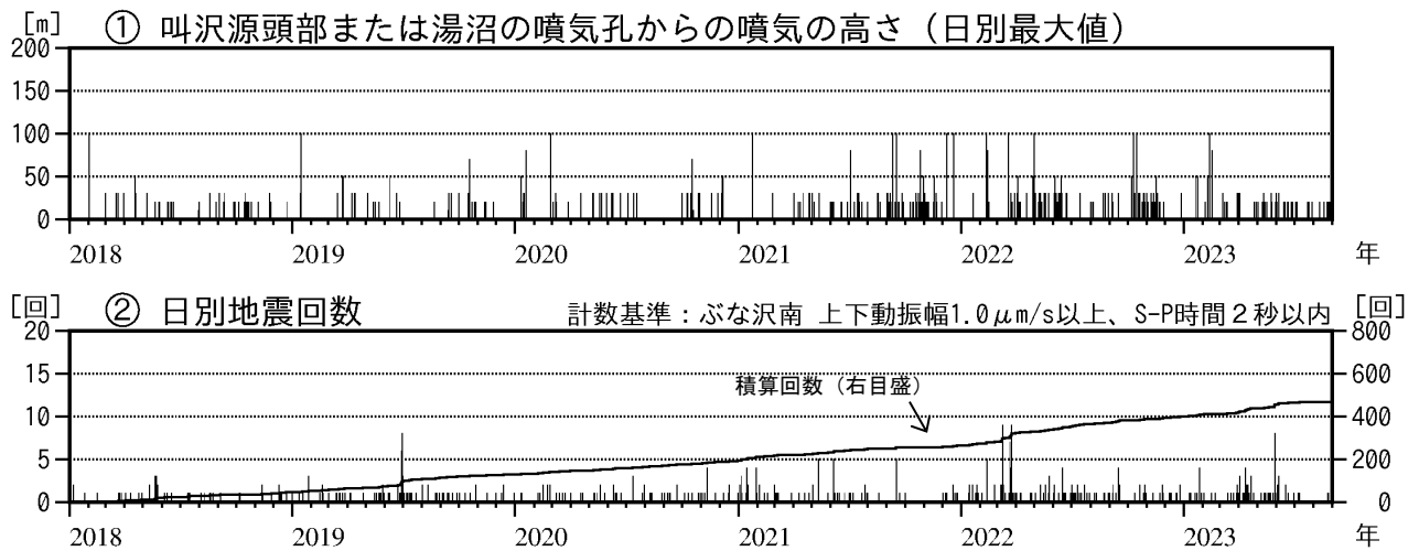
図3 秋田焼山 火山活動経過図（2018年1月～2023年8月）
