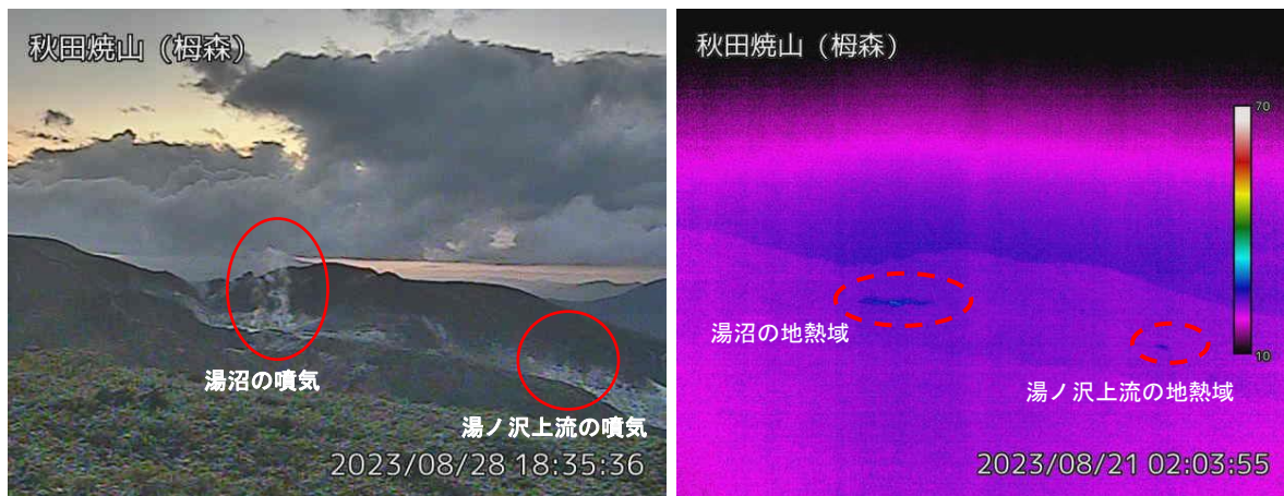
図2 秋田焼山 湯沼と湯ノ沢上流の状況（8月28日）と地表面温度分布（8月21日）
