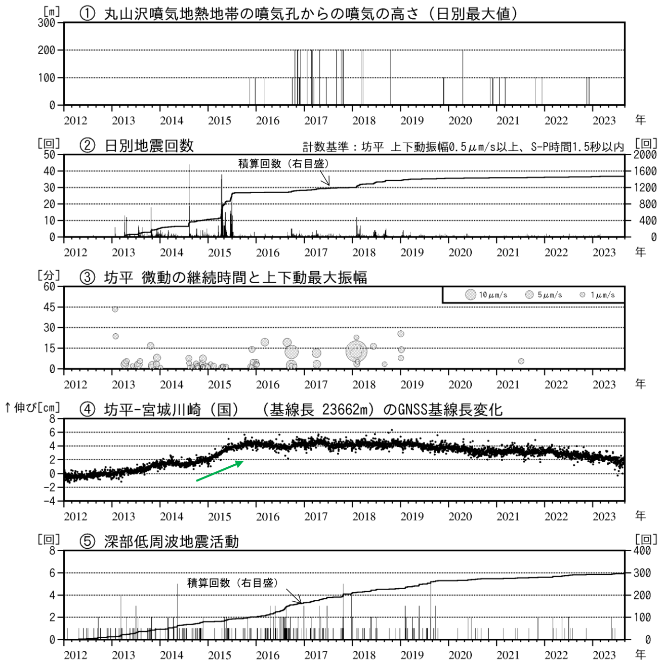
図4 蔵王山 火山活動経過図（2012年1月～2023年8月）
