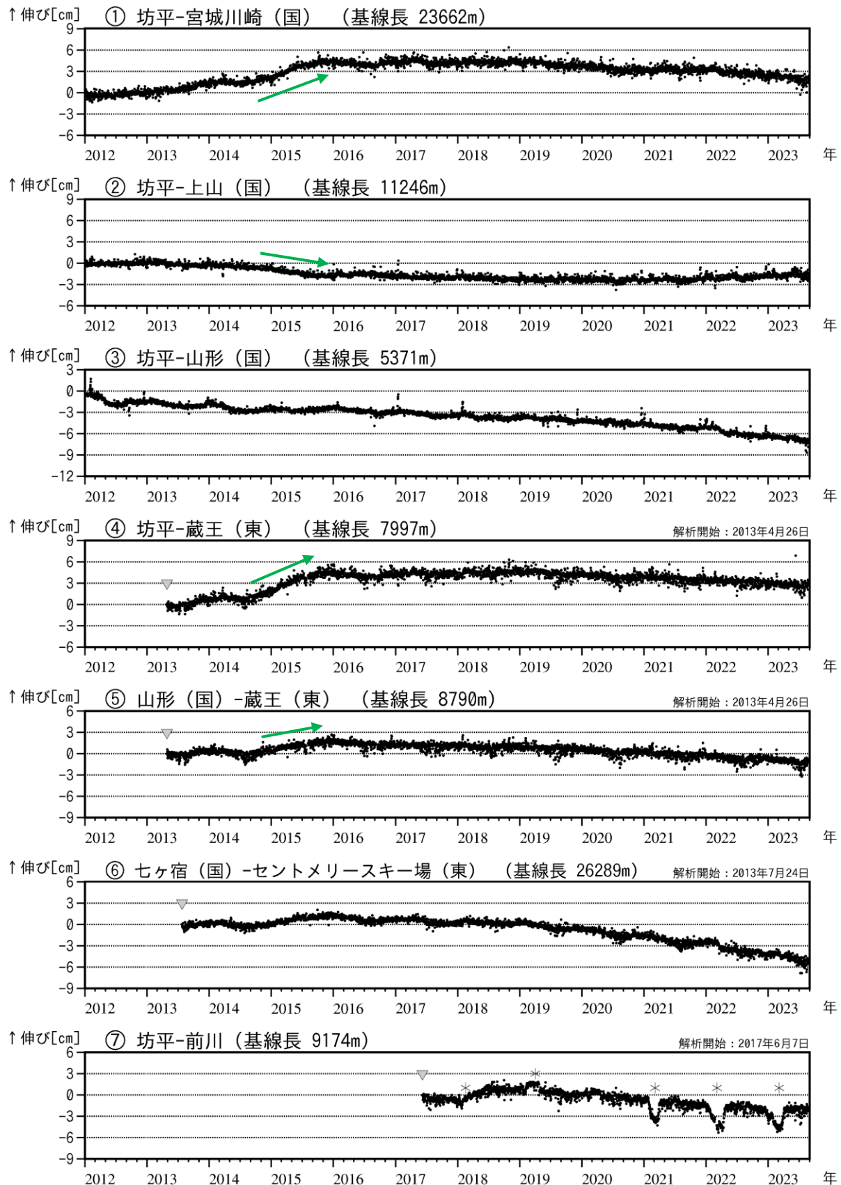
図5 蔵王山 GNSS 基線長変化図（2012年1月～2023年8月）
