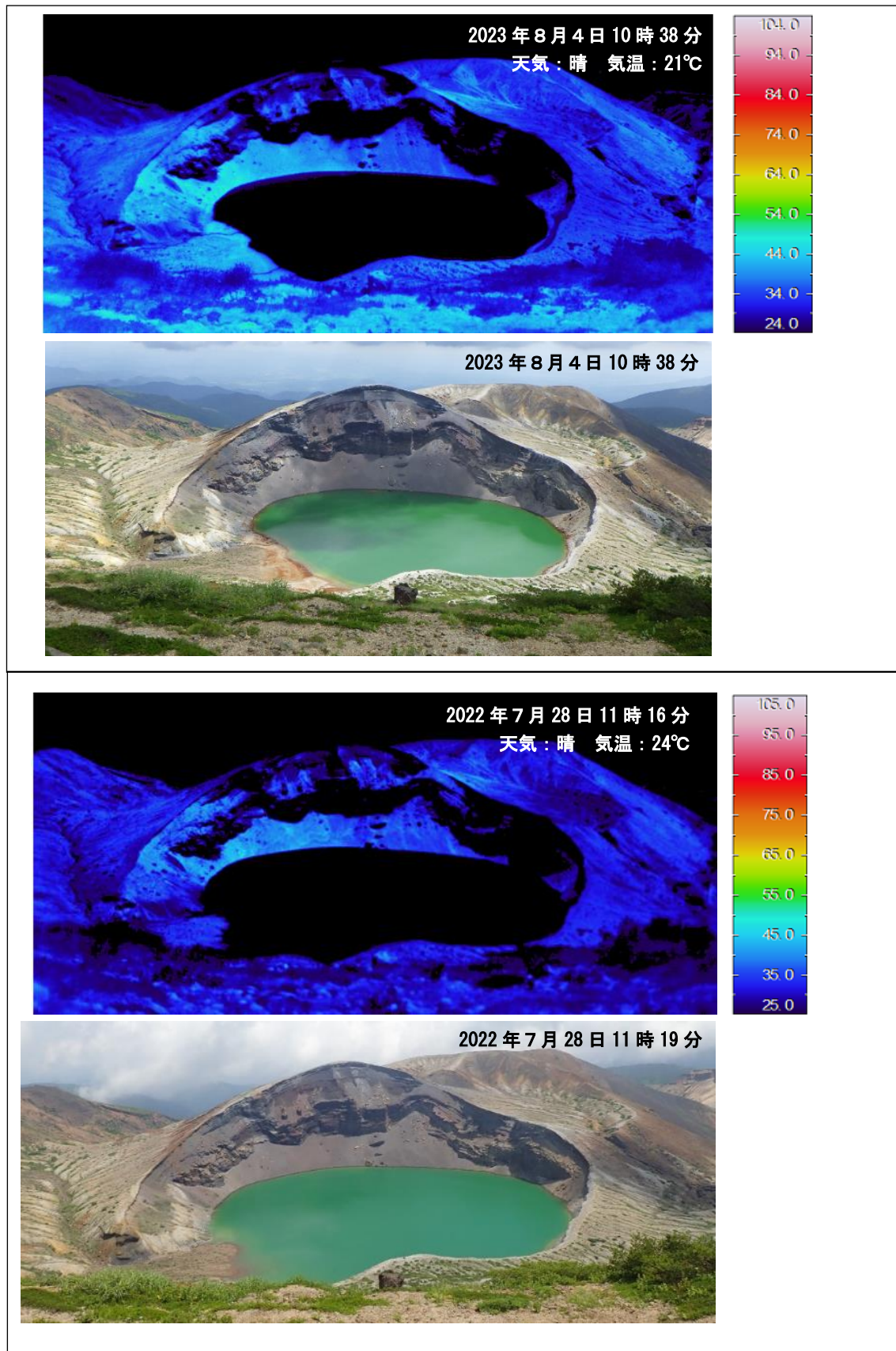
図3 蔵王山 西から撮影した御釜周辺の状態（下段）と地表面温度分布（上段）
