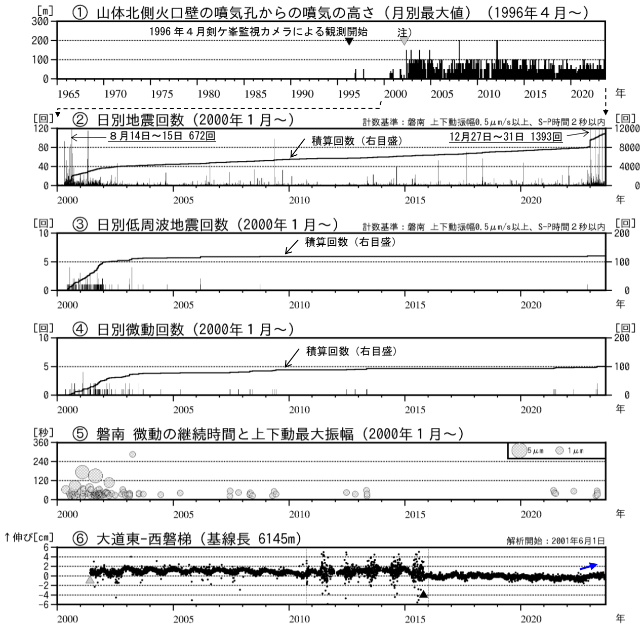
図3 磐梯山 火山活動経過図（1965年7月～2023年8月）
