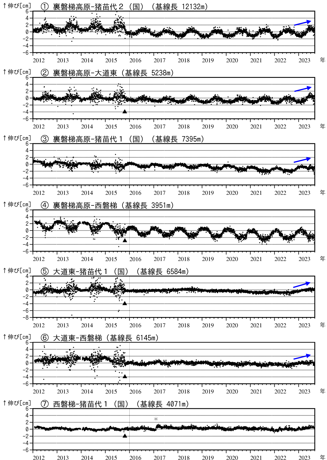
図6 磐梯山 GNSS 基線長変化図 (2012年1月～2023年8月)
