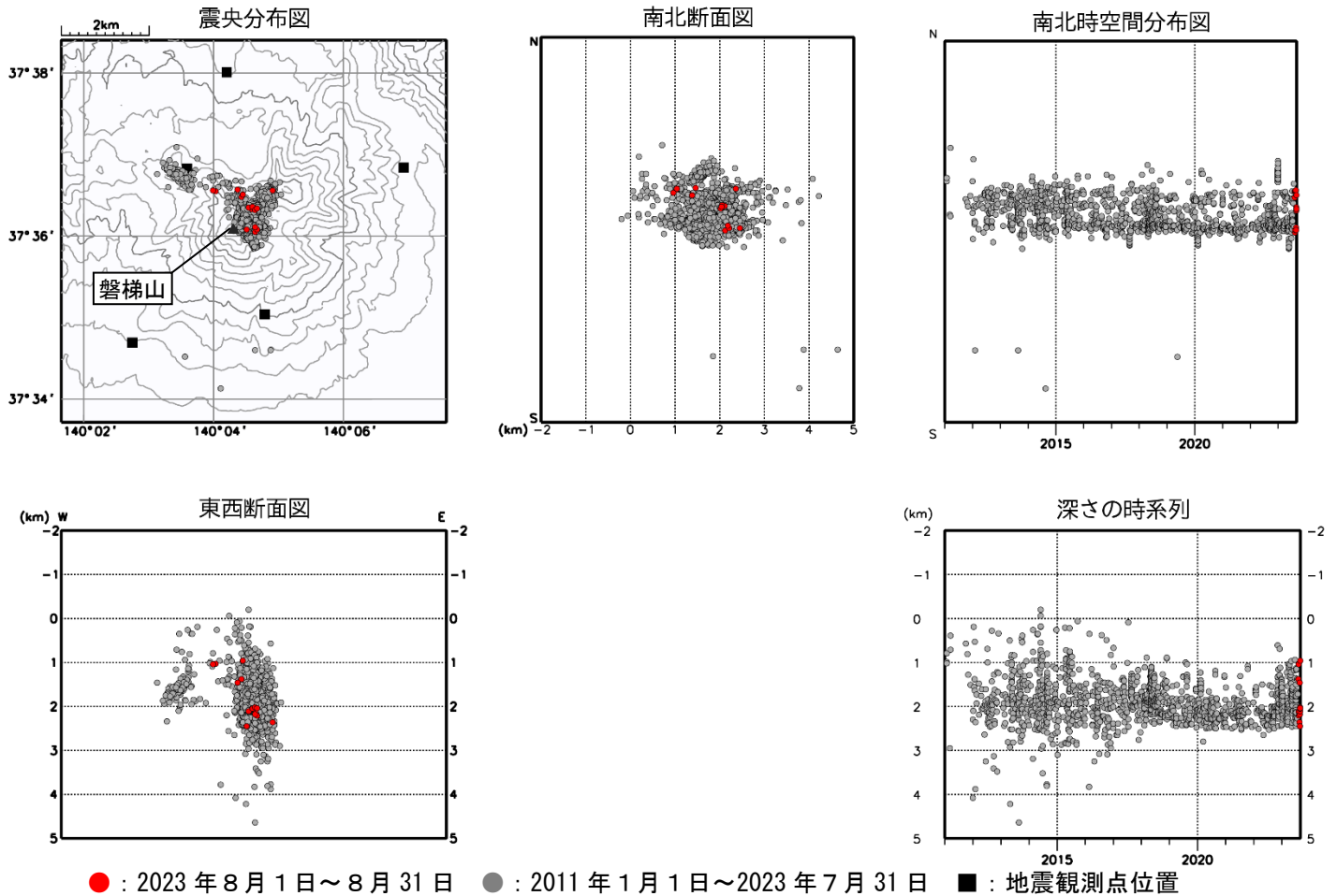
図5 磐梯山 震源分布図（2011年1月～2023年8月）
