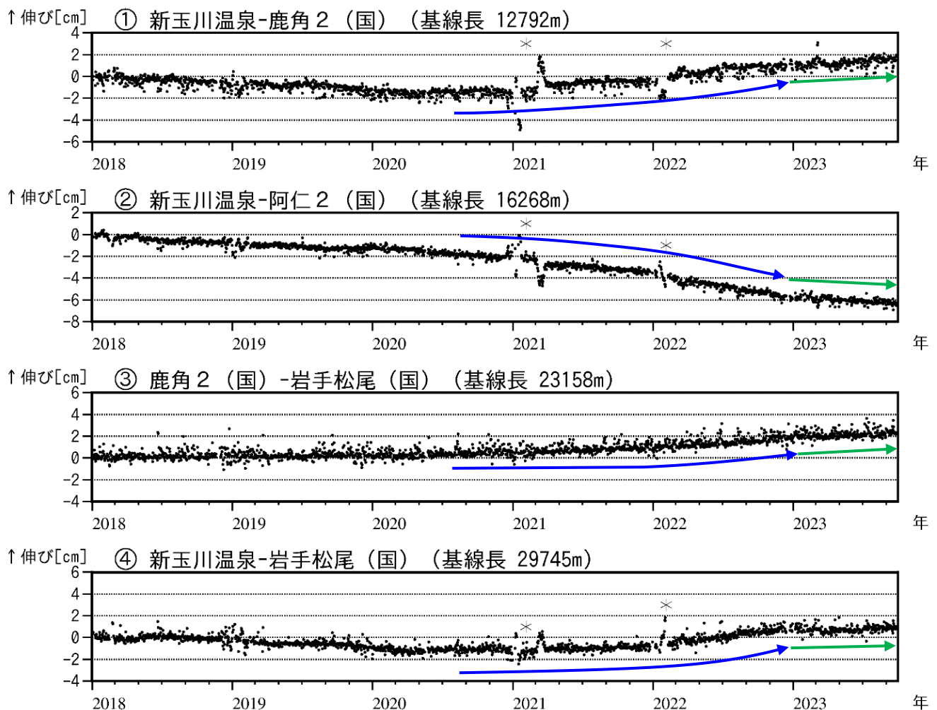
図4 秋田焼山 GNSS 基線長変化図（2018年1月～2023年9月）
