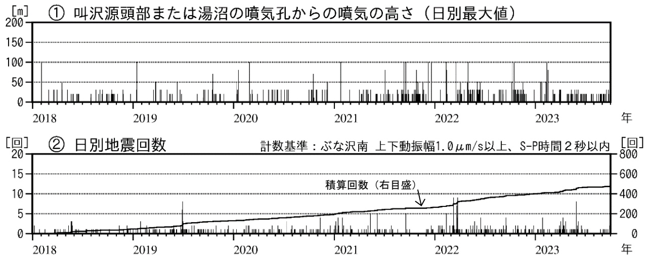
図3 秋田焼山 火山活動経過図（2018年1月～2023年9月）
