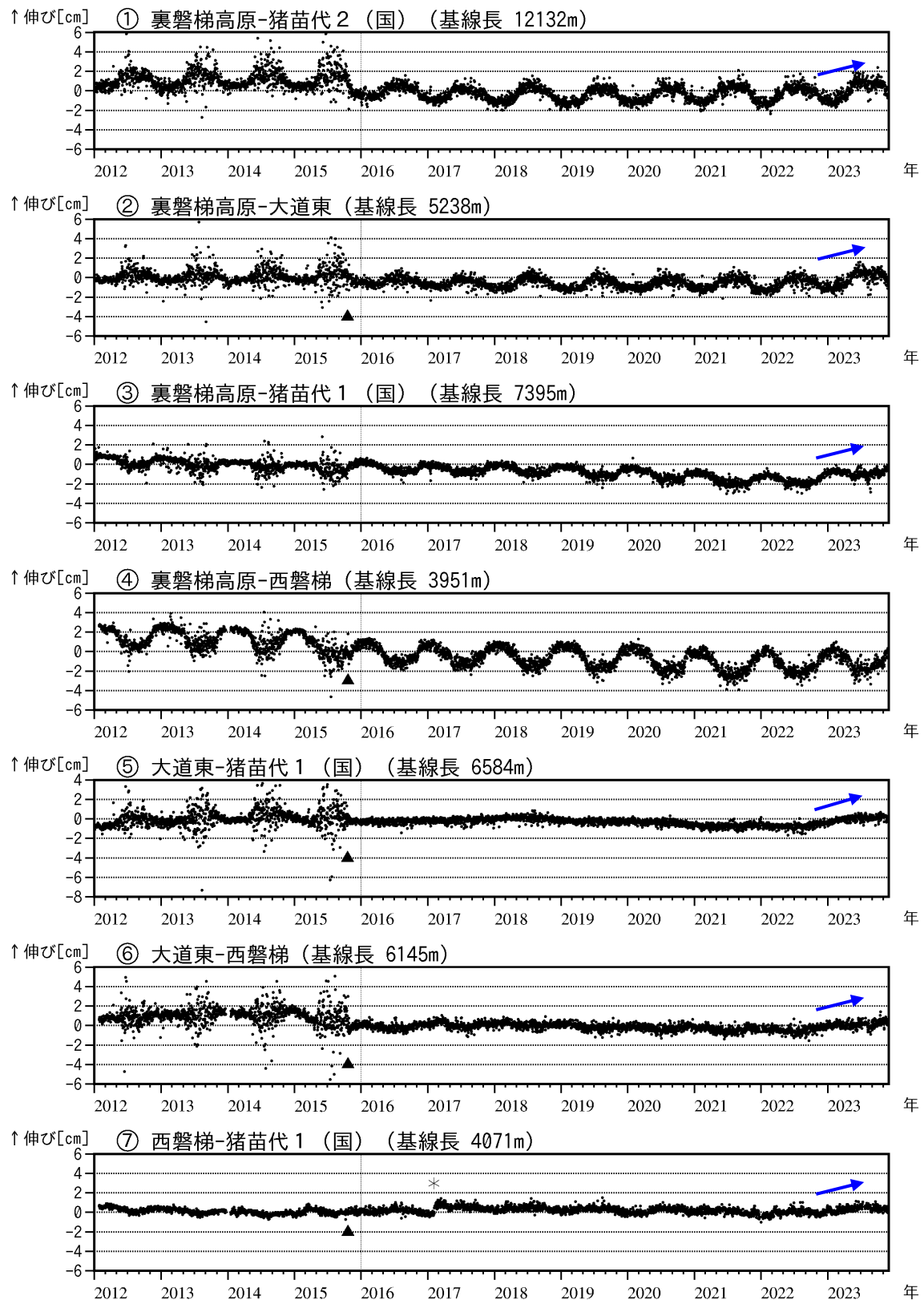
図7 磐梯山 GNSS 基線長変化図（2012年1月～2023年11月）
