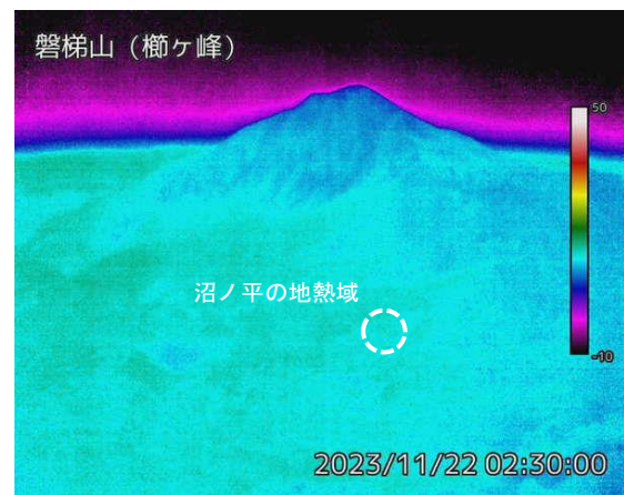
図2 磐梯山 沼ノ平周辺の状況（11月12日）と地表面温度分布（11月22日）
