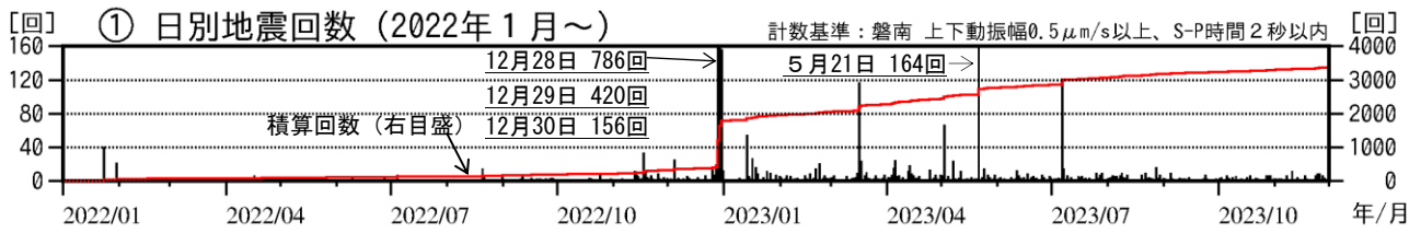
図5 磐梯山 地震回数（2022年1月～2023年11月）
