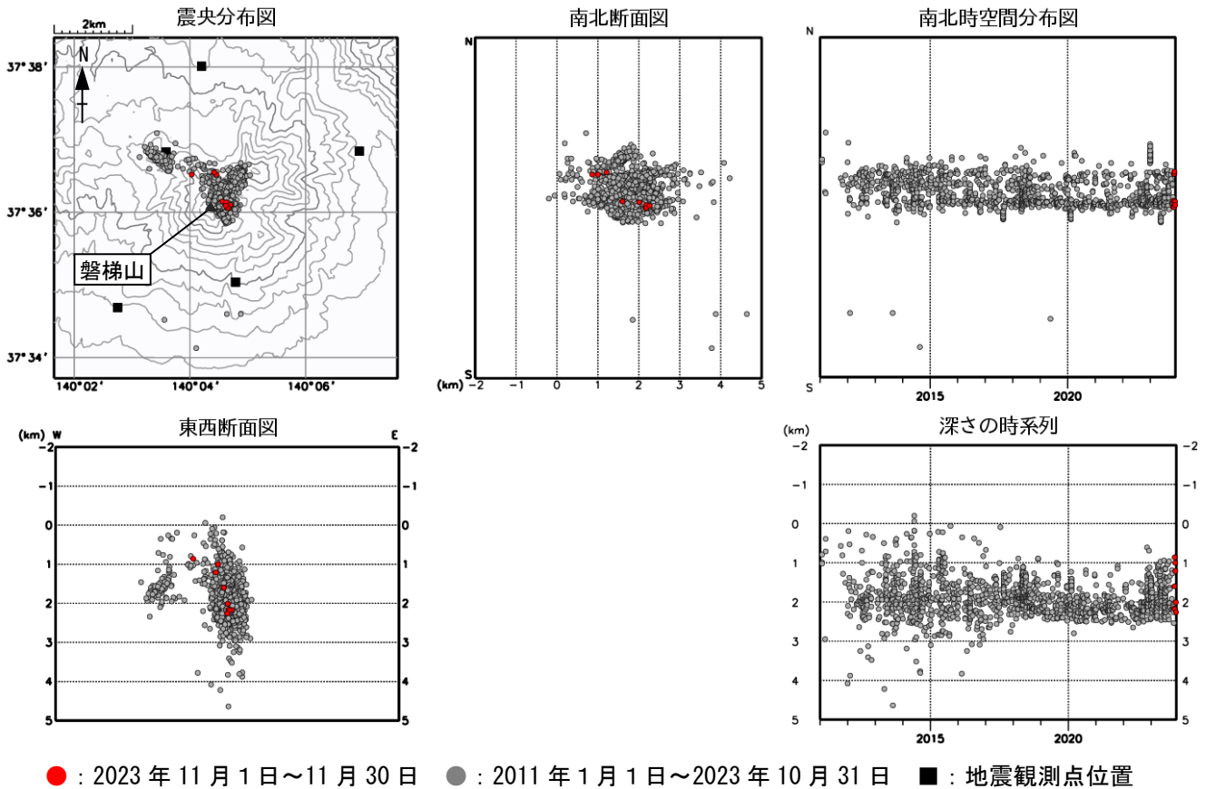
図6 磐梯山 震源分布図（2011年1月～2023年11月）
