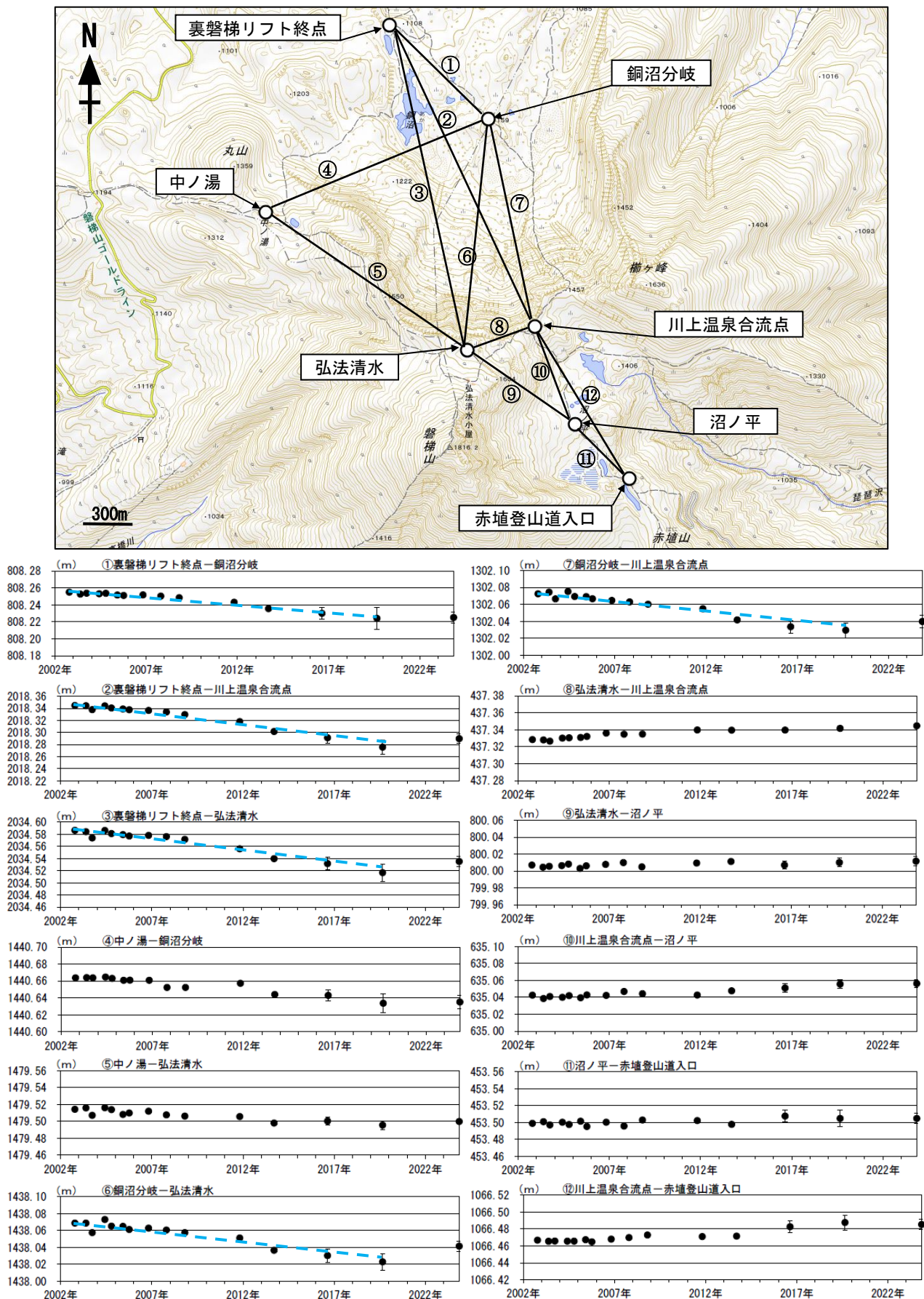
図3 磐梯山 GNSS 繰り返し観測結果 (2002 年 1 月～2023 年 11 月)
