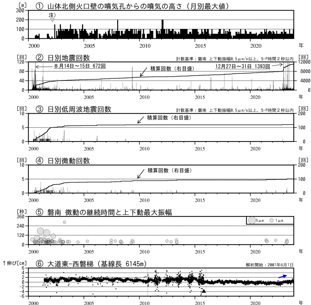
図4 磐梯山 火山活動経過図（2000年1月～2023年11月）
