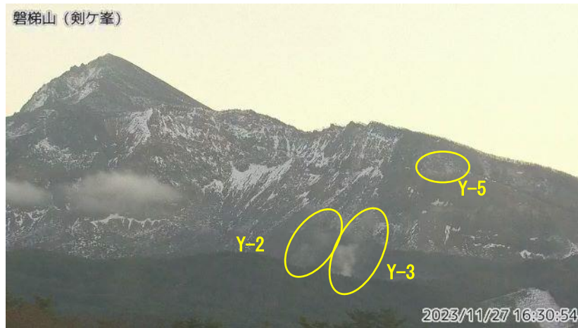
図1 磐梯山 山体北側火口壁の噴気の状態（11月27日）
