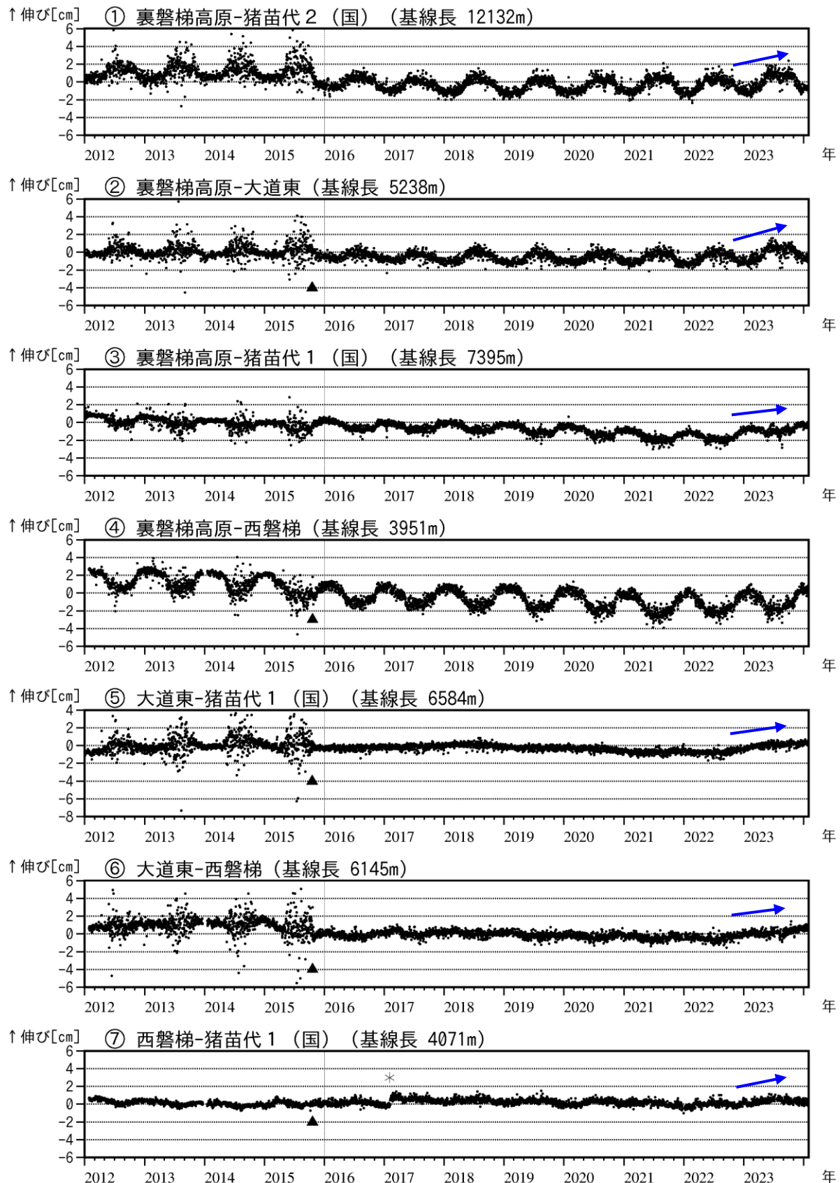
図6 磐梯山 GNSS 基線長変化図（2012年1月～2024年1月）
