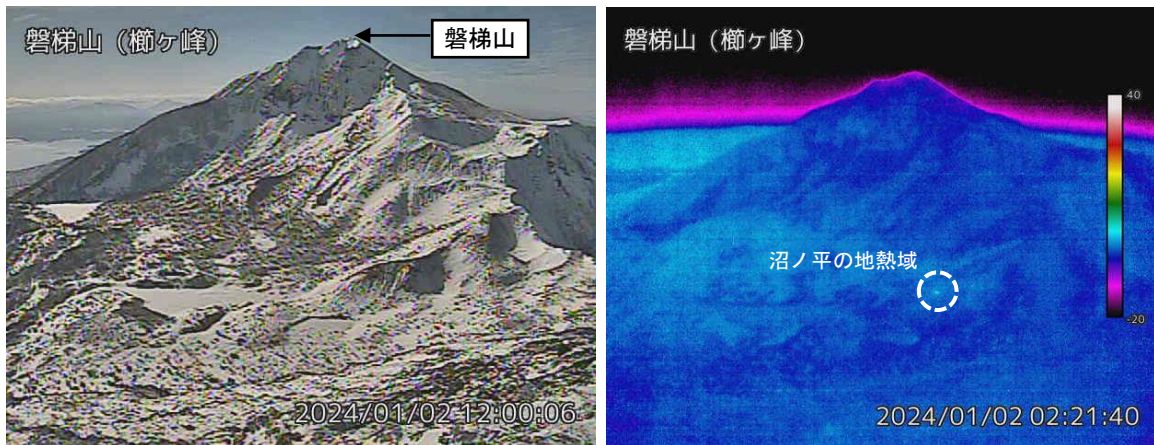
図2 磐梯山 沼ノ平周辺の状況と地表面温度分布（1月2日）
