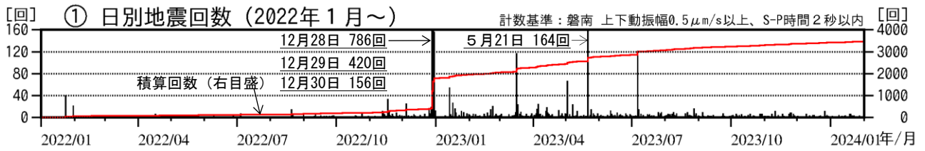
図4 磐梯山 地震回数（2022年1月～2024年1月）
