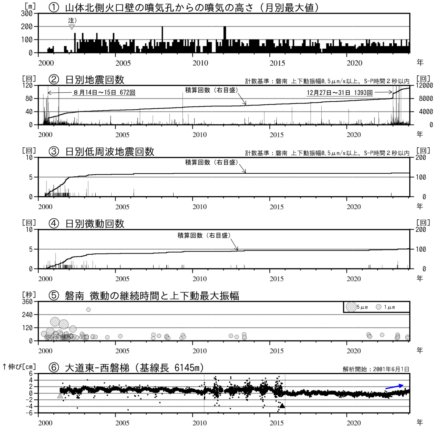
図3 磐梯山 火山活動経過図（2000年1月～2024年1月）
