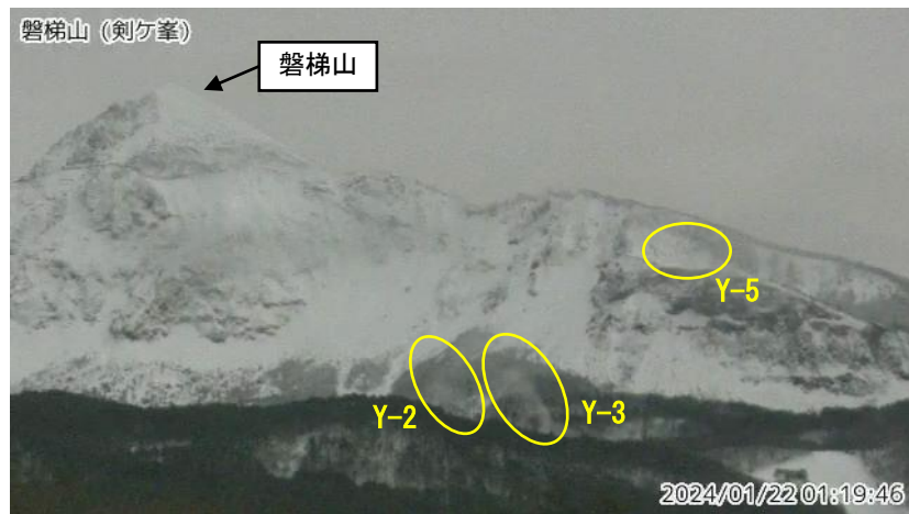
図1 磐梯山 山体北側火口壁の噴気の状態（1月22日）
