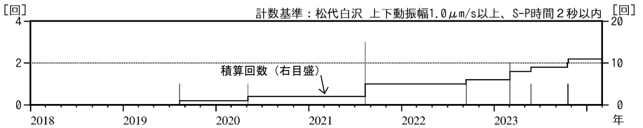
図2 岩木山 日別地震回数（2018年1月～2024年2月）
