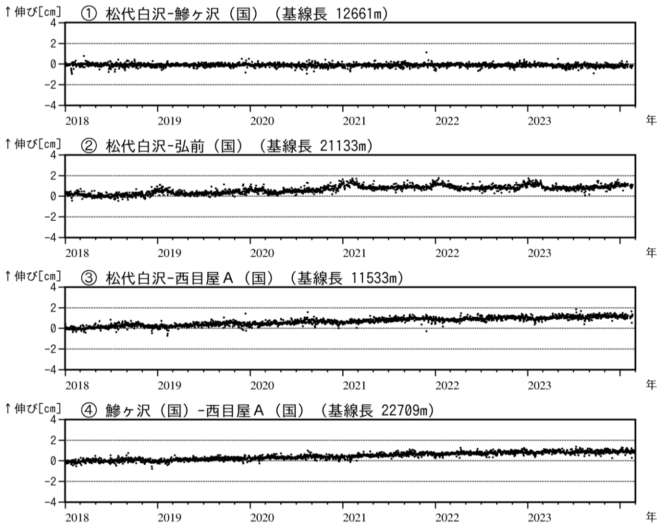
図3 岩木山 GNSS 基線長変化図（2018年1月～2024年2月）
