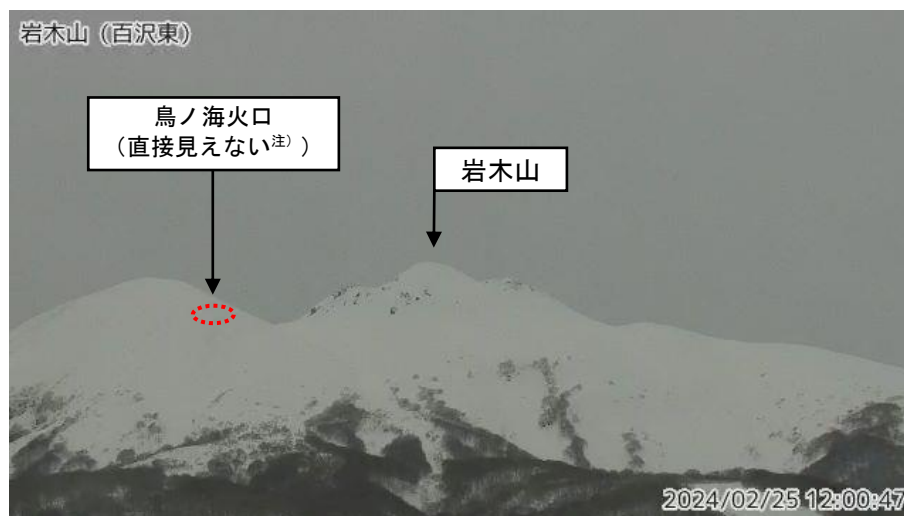
図1 岩木山 山頂部の状況（2月25日）
