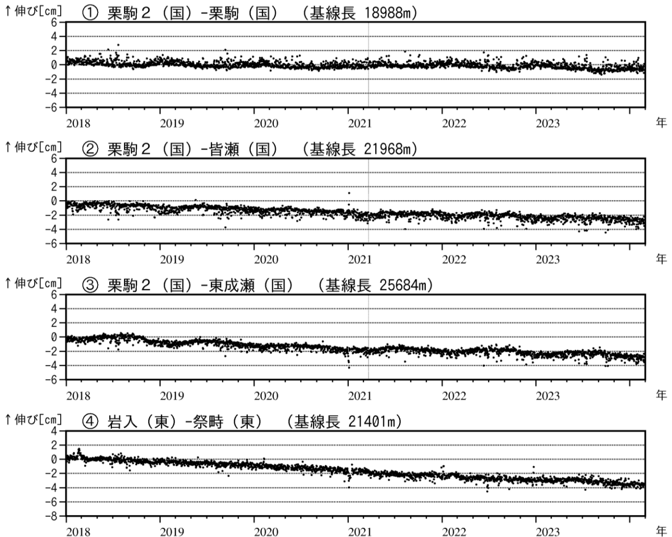
図3 栗駒山 GNSS 基線長変化図（2018年1月～2024年2月）
