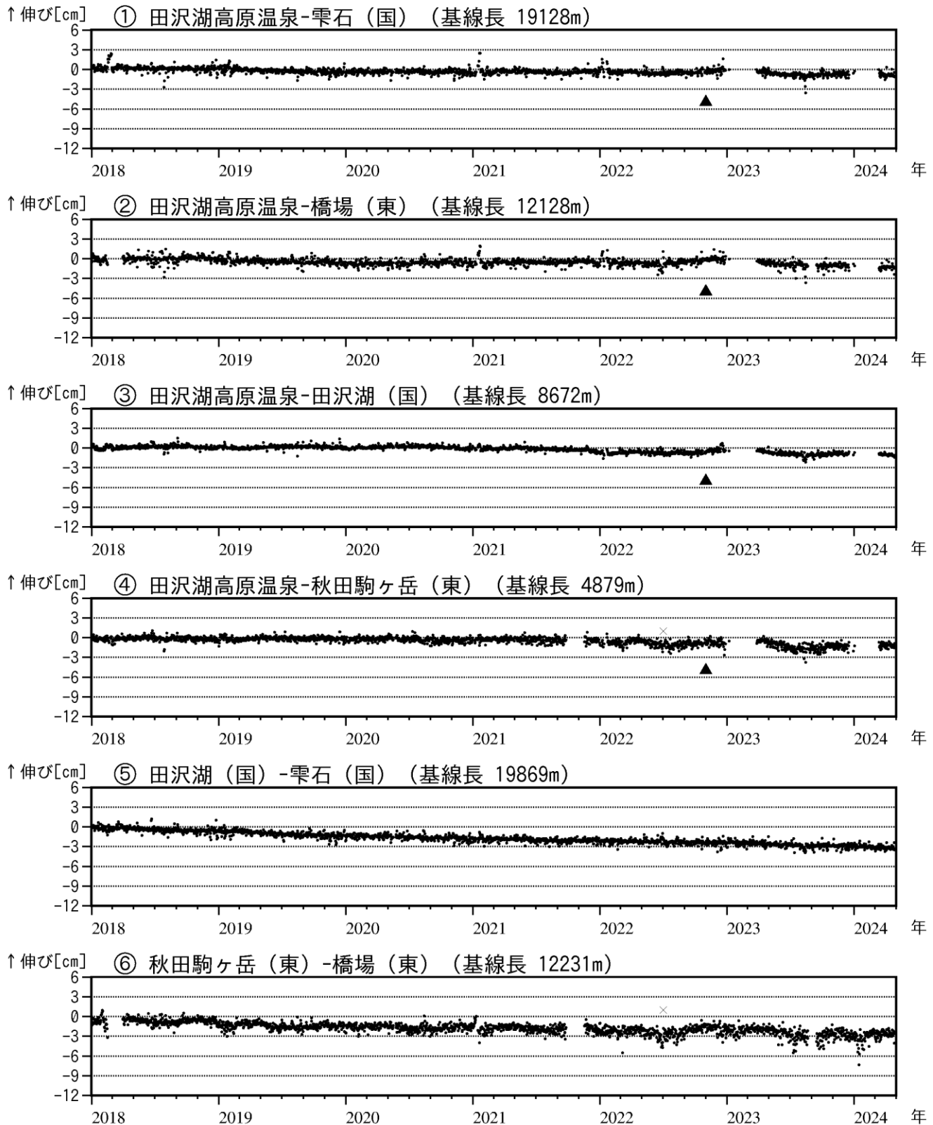
図5 秋田駒ヶ岳 GNSS 基線長変化図（2018年1月～2024年4月）
