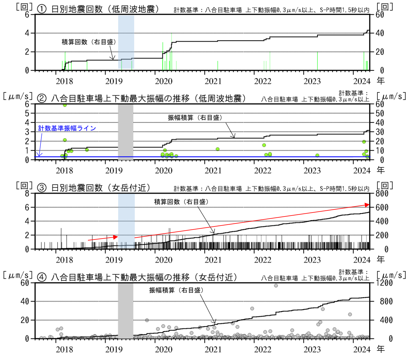
図3 秋田駒ヶ岳 低周波地震及び女岳付近の日別回数と最大振幅（2017年8月～2024年4月）
