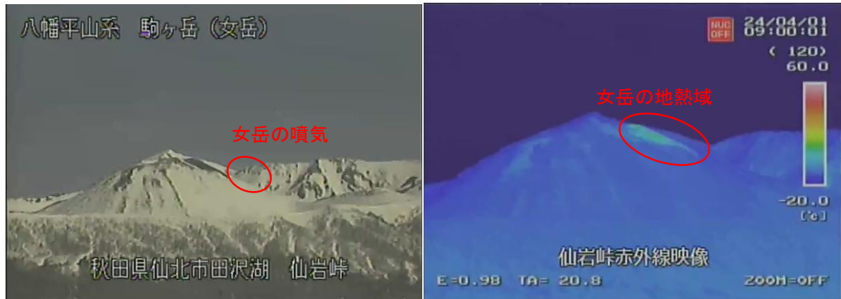
図1 秋田駒ヶ岳 女岳周辺の状況と地表面温度分布の状況（4月1日）
