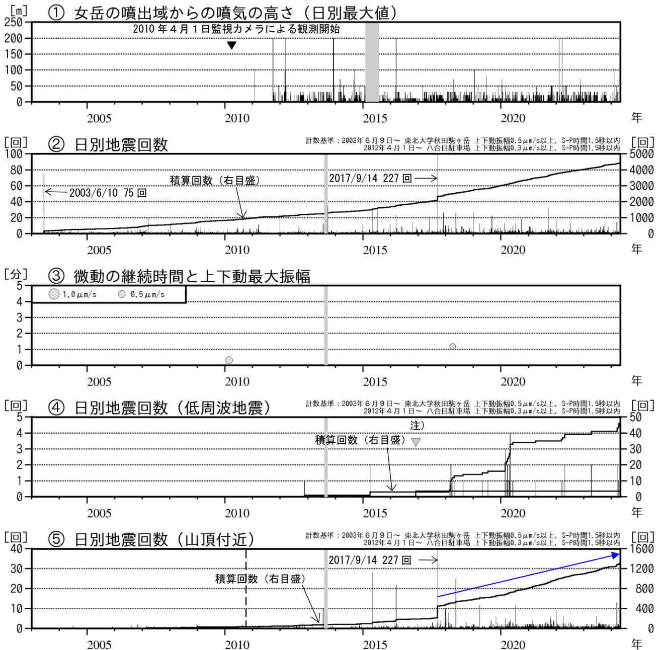
図2 秋田駒ヶ岳 火山活動経過図（2003年6月～2024年4月）
