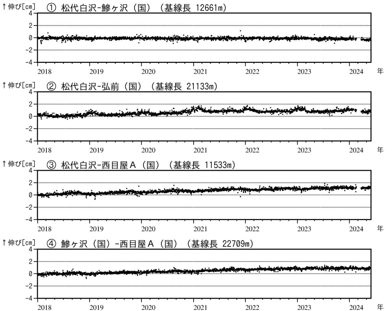
図3 岩木山 GNSS 基線長変化図（2018年1月～2024年5月）
