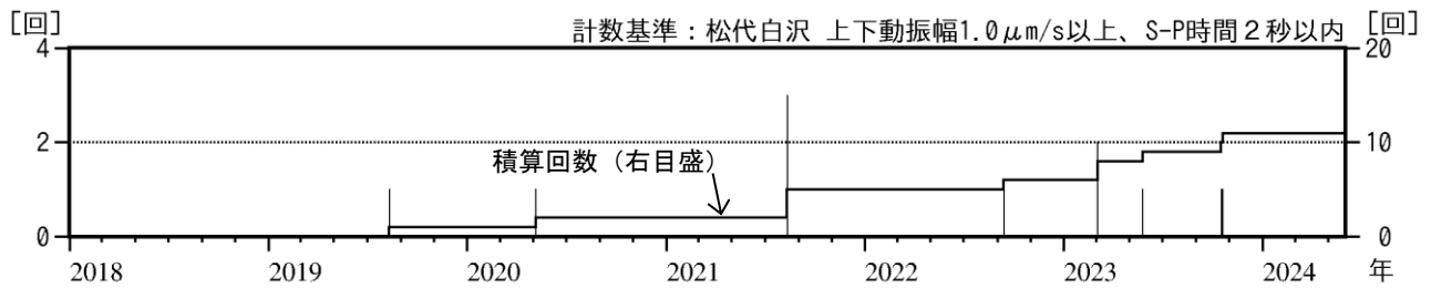
図2 岩木山 日別地震回数（2018年1月～2024年5月）
