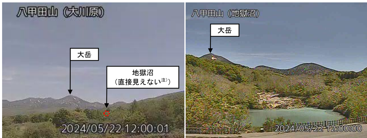
図1 八甲田山 山頂部及び地獄沼周辺の状況（5月22日）
