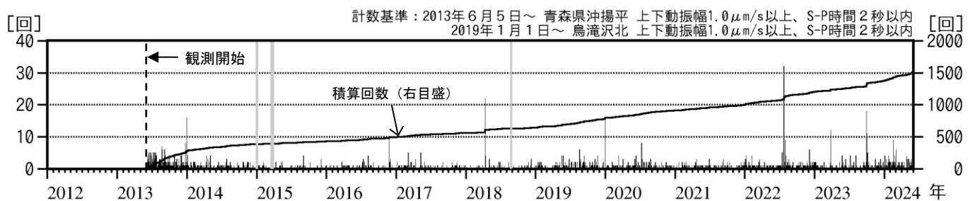
図2 八甲田山 日別地震回数（2013年6月～2024年5月）
