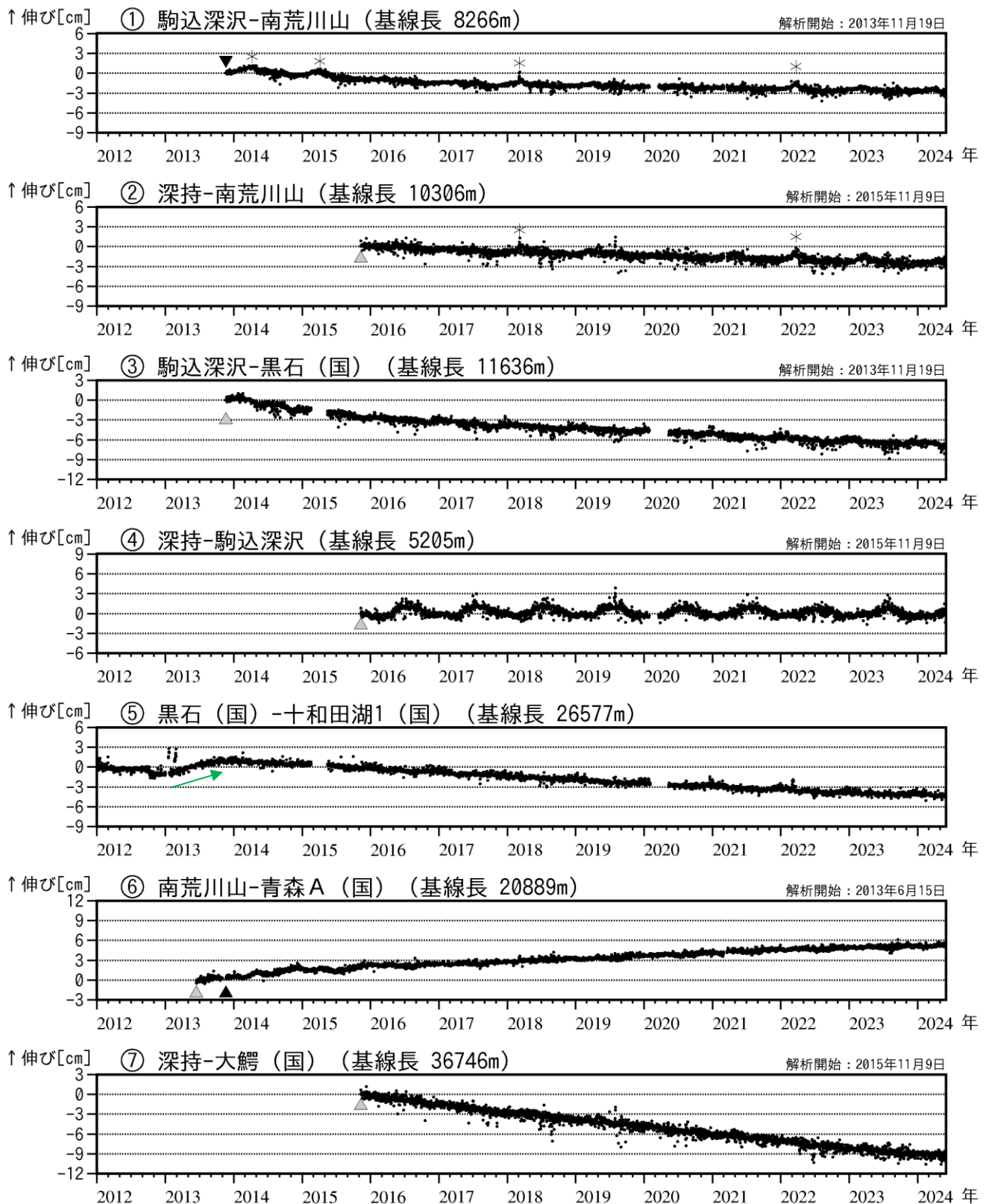
図3 八甲田山 GNSS 基線長変化図（2012年1月～2024年5月）
