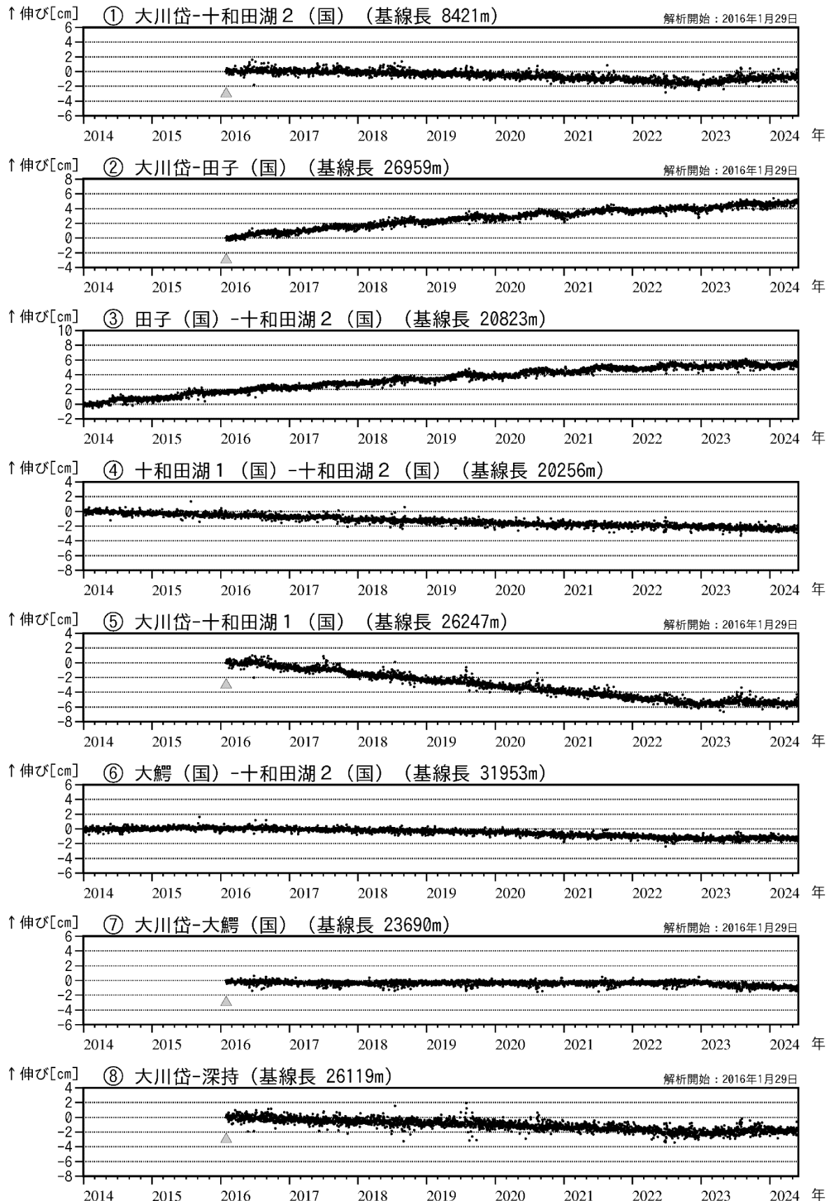
図3 十和田 GNSS 基線長変化図（2014年1月～2024年5月）
