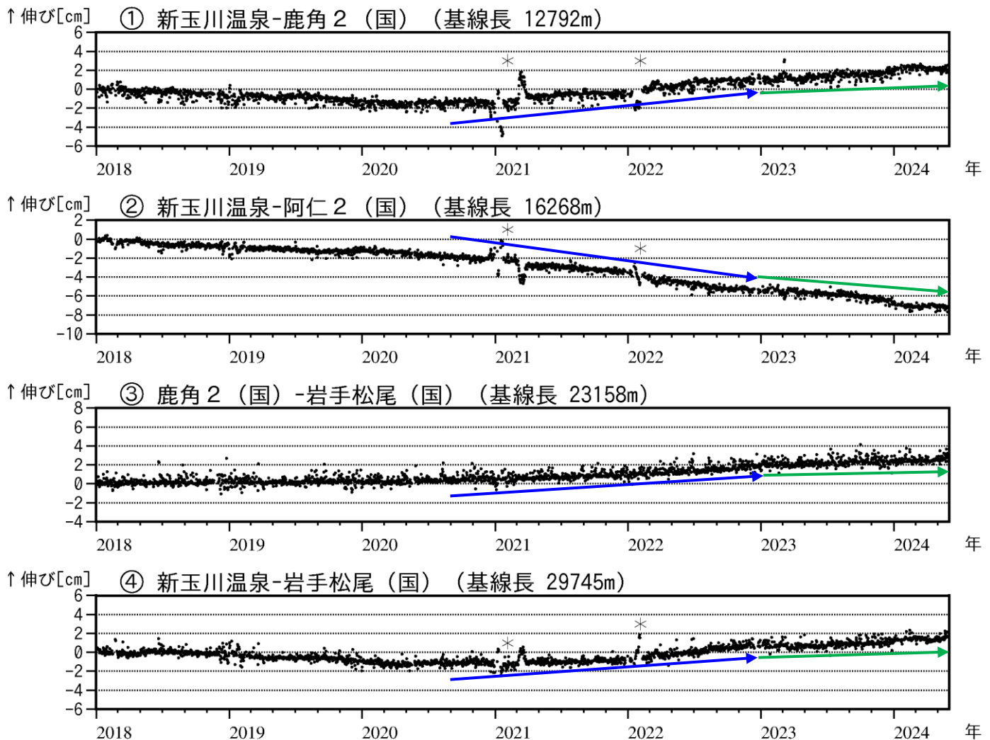
図4 秋田焼山 GNSS 基線長変化図（2018年1月～2024年5月）
