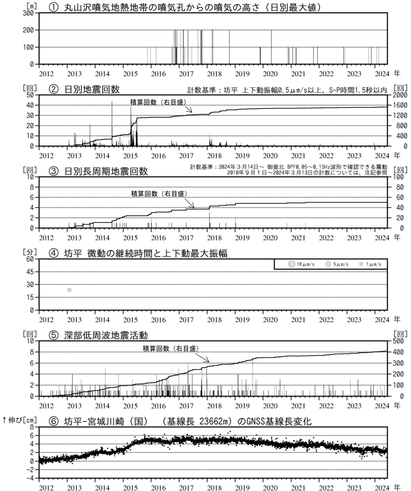
図2 蔵王山 火山活動経過図（2012年1月～2024年5月）
