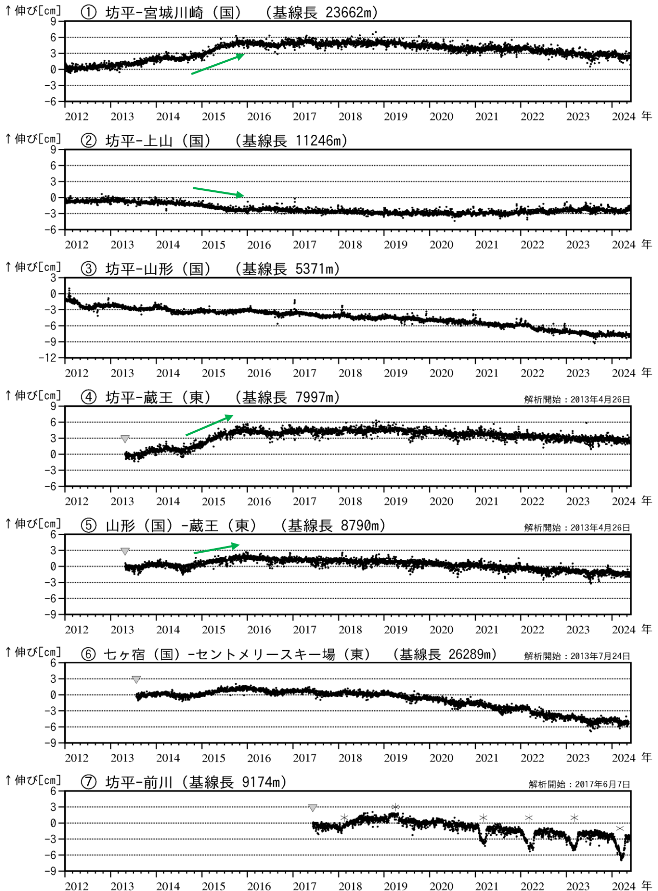
図3 蔵王山 GNSS 基線長変化図（2012年1月～2024年5月）
