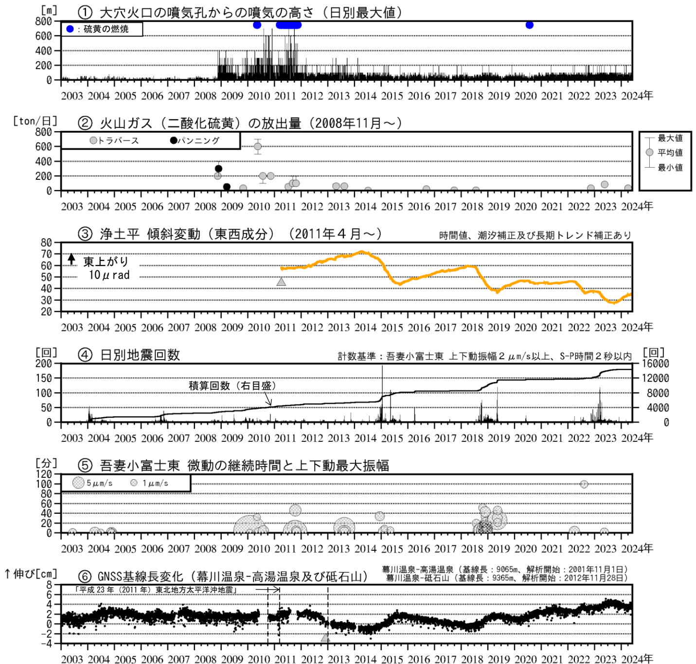
図2 吾妻山 中期的な火山活動の経過（2003年1月～2024年5月）
