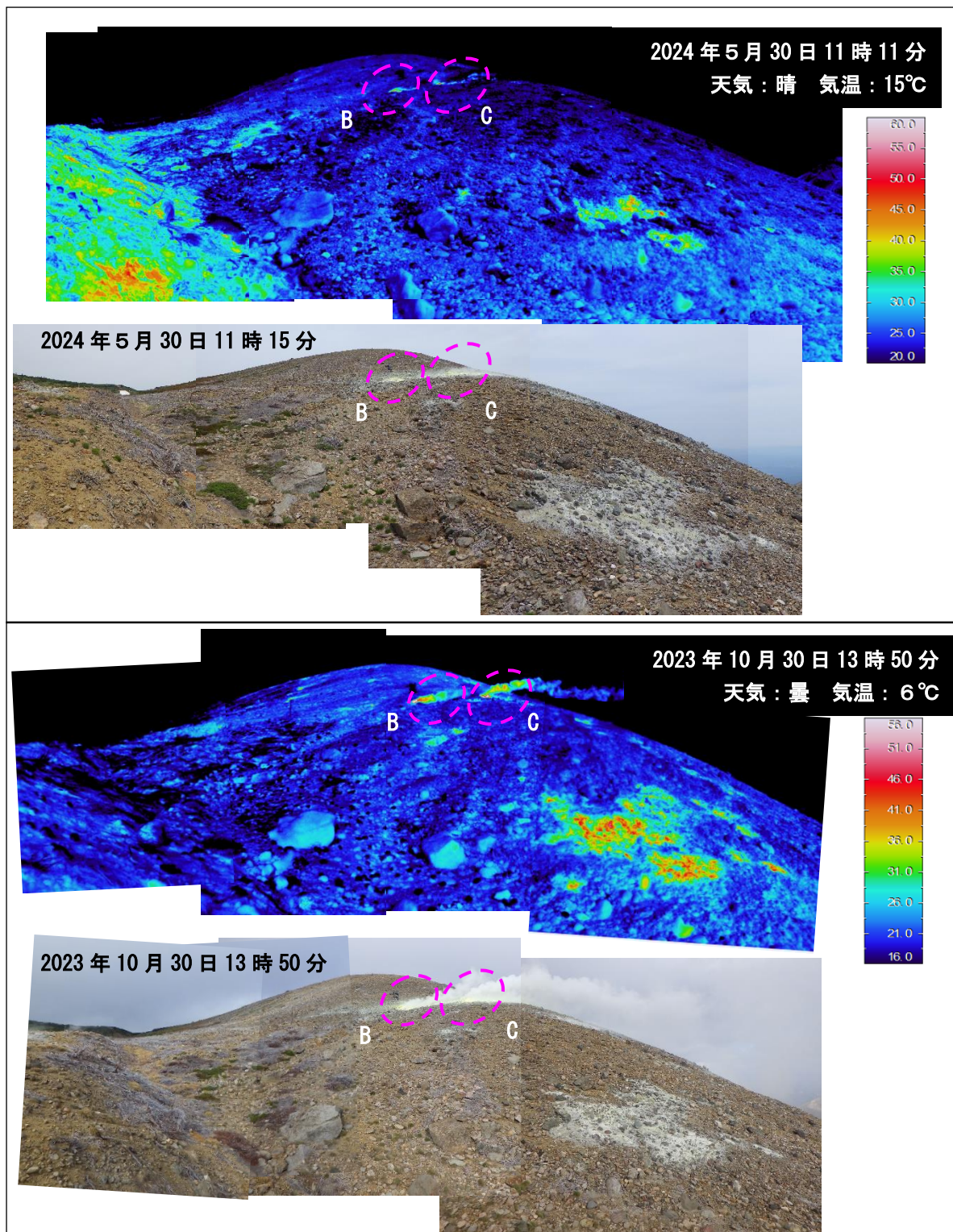
図10 吾妻山 大穴火口北西の状況（下）と地表面温度分布（上）
