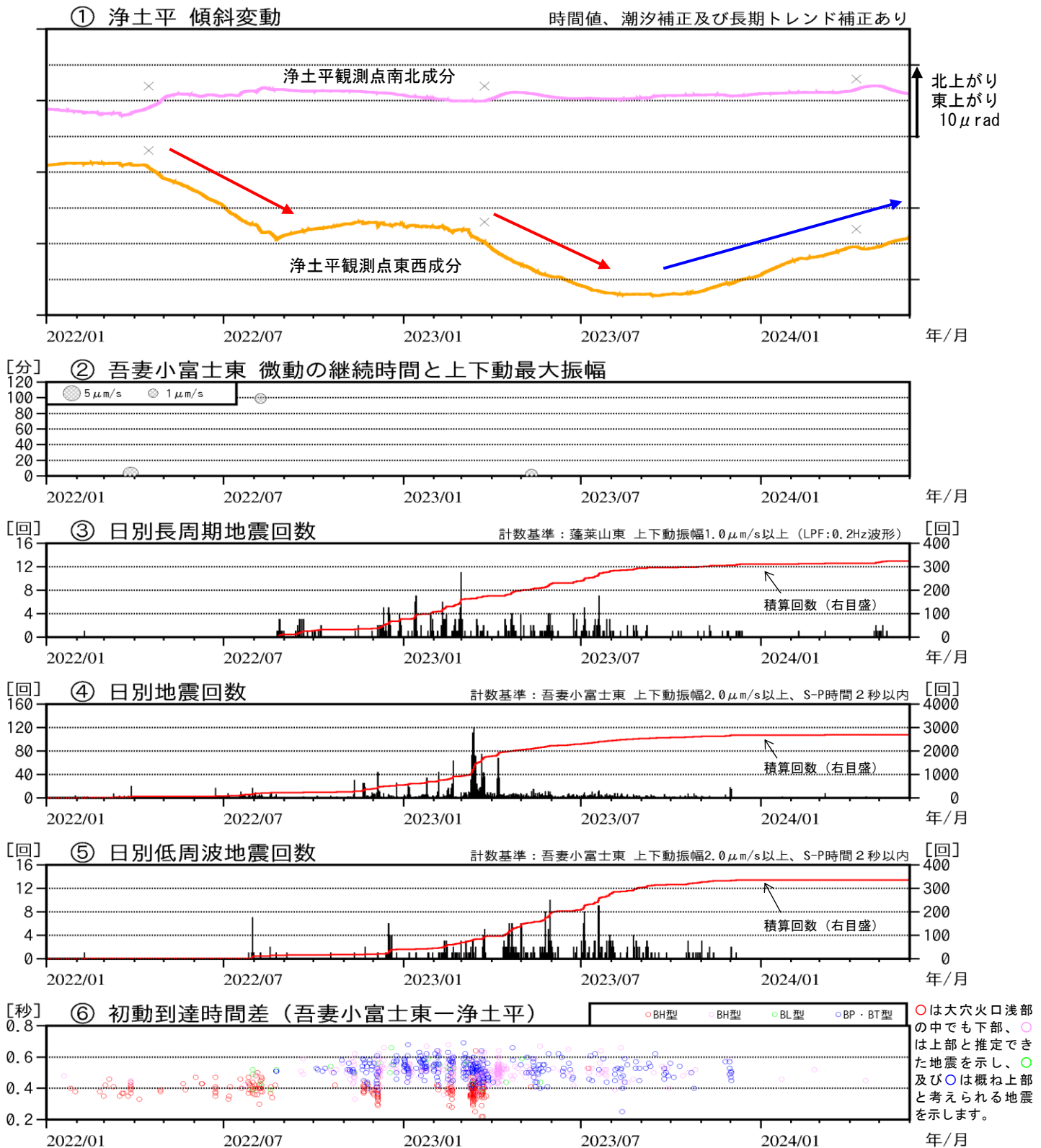
図3 吾妻山 火山活動経過図（2022年1月～2024年5月）
