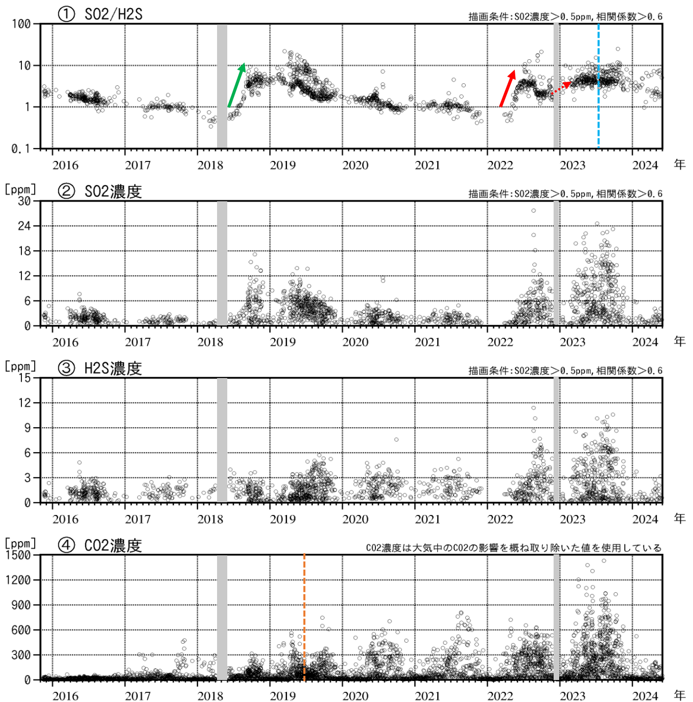
図12 吾妻山 火山ガス観測装置による観測（2015年11月～2024年5月）
