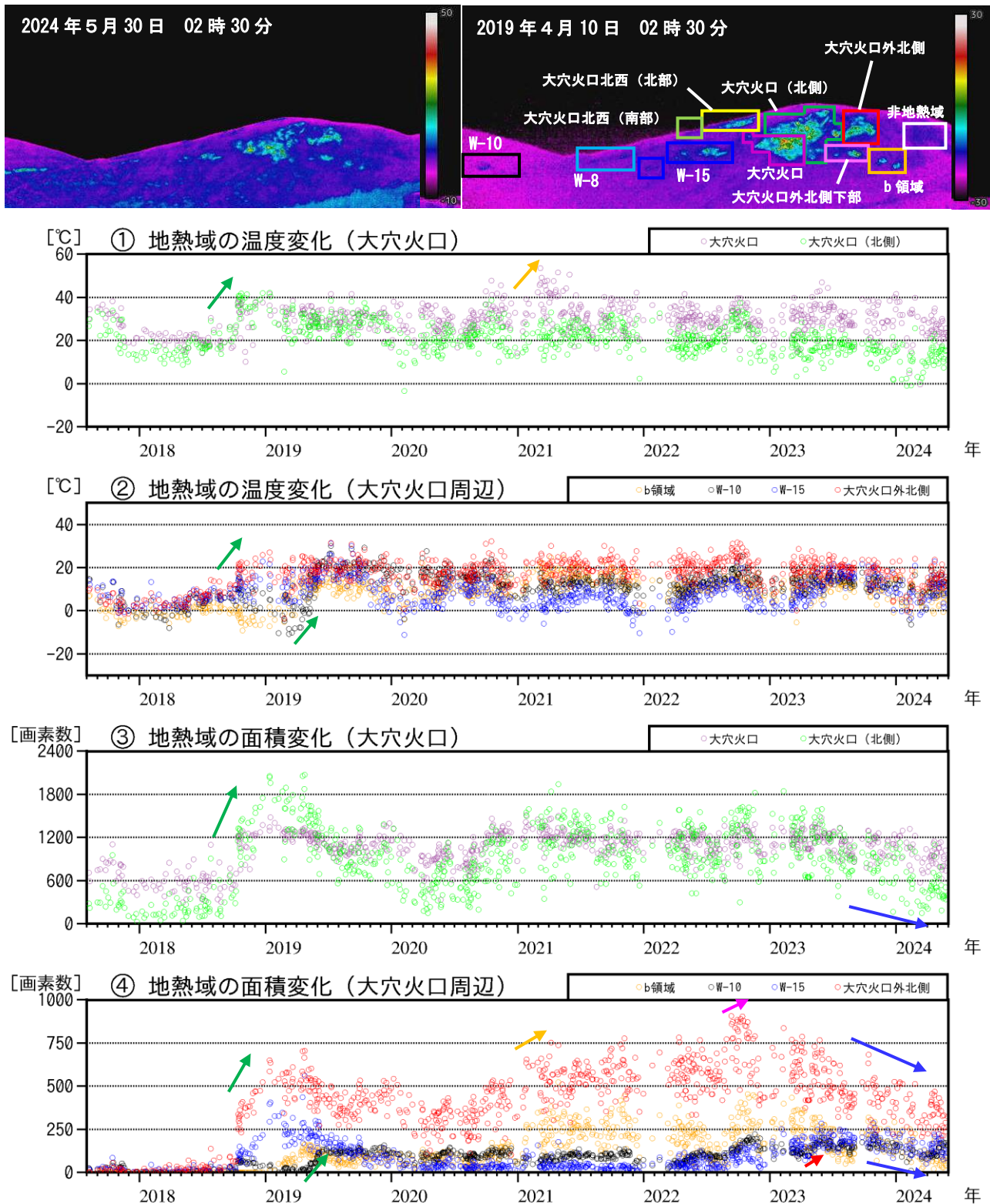
図5 吾妻山 監視カメラによる大穴火口周辺の地熱域の経過（2017年8月～2024年5月）
