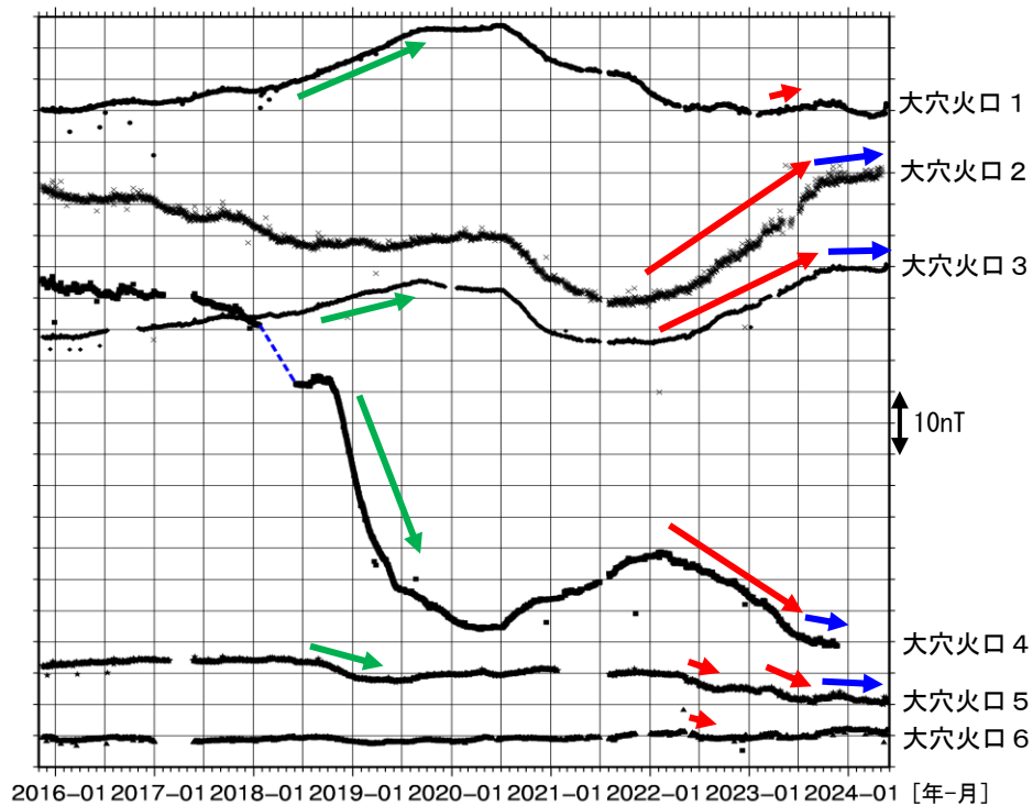
図 13 吾妻山 全磁力連続観測点の全磁力値変化（2015 年 11 月～2024 年 5 月）
