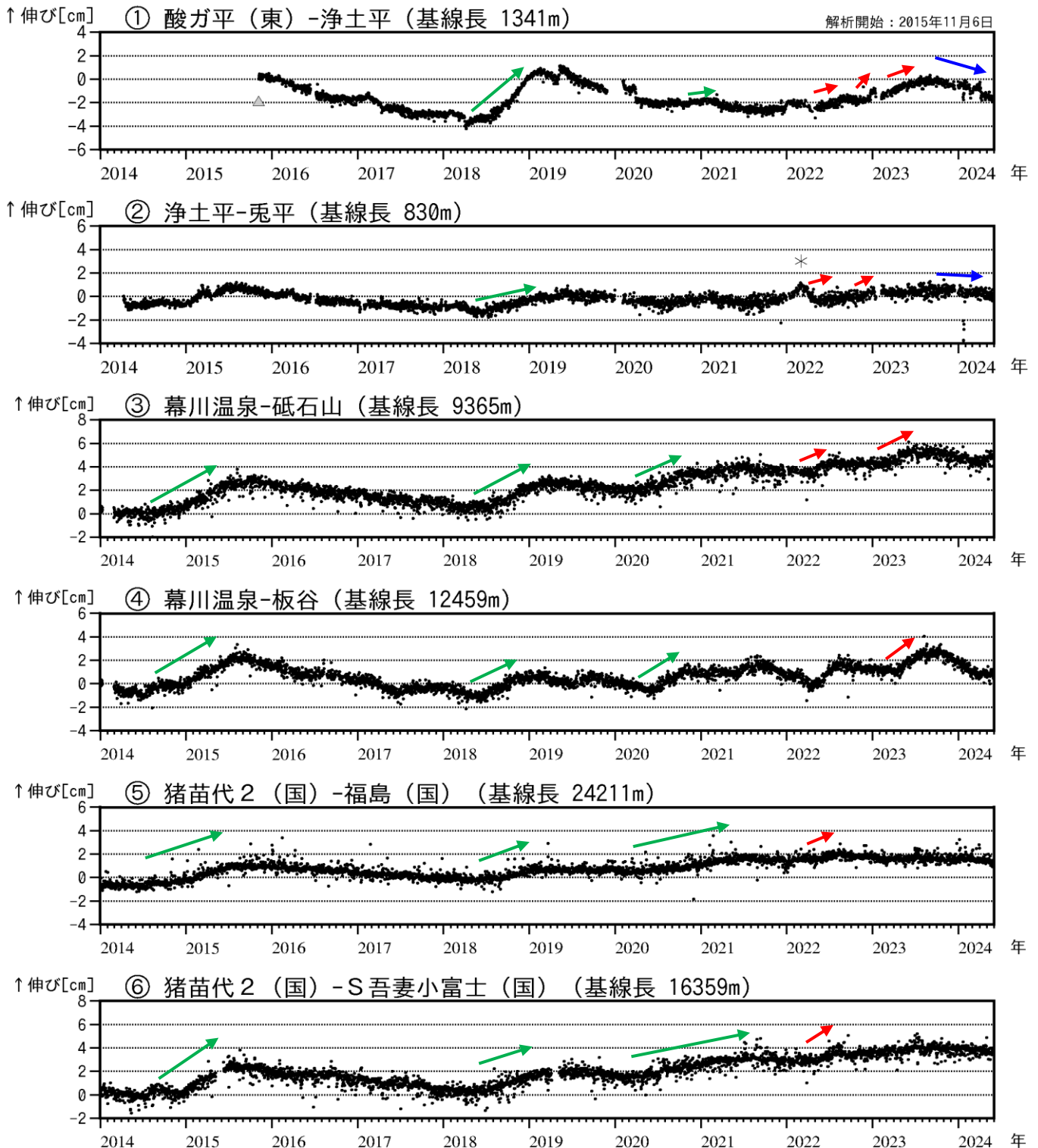
図4 吾妻山 吾妻山浅部・深部の地殻変動(2014年1月~2024年5月)
