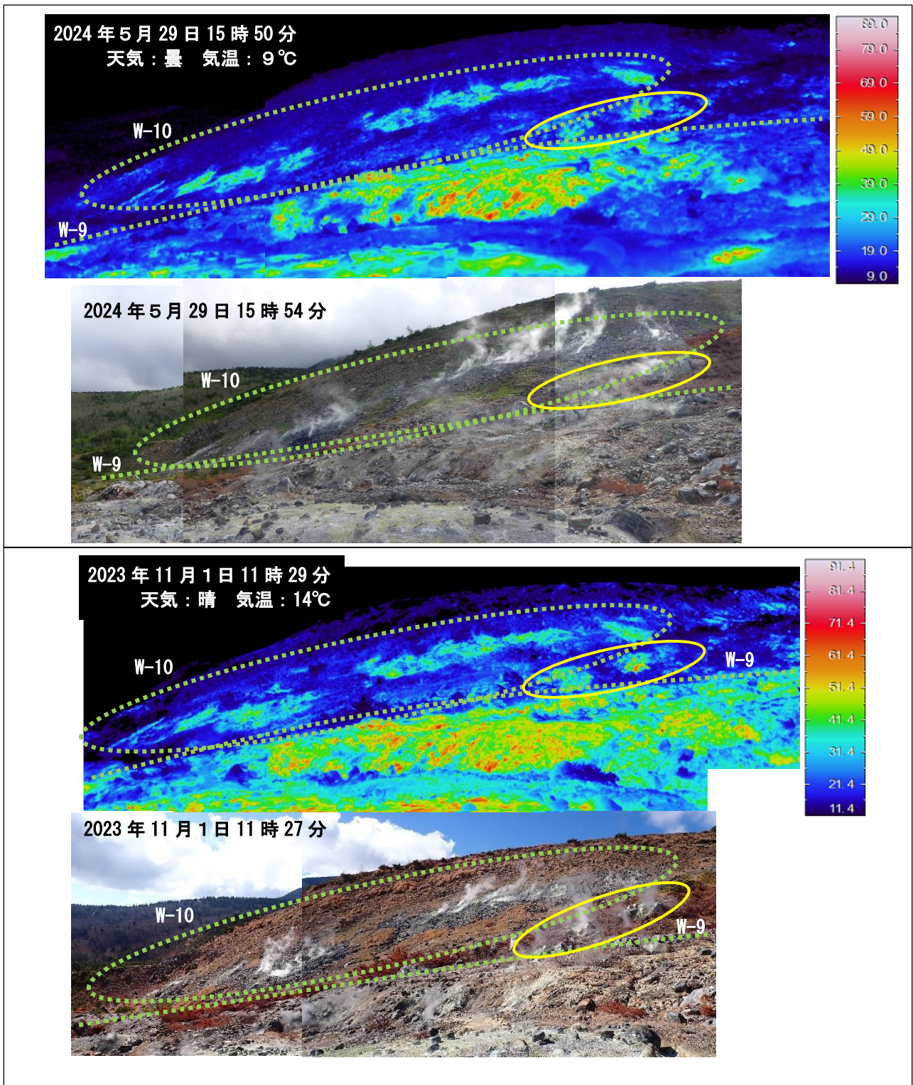
図11 吾妻山 八幡焼の状況（下）と地表面温度分布（上）
