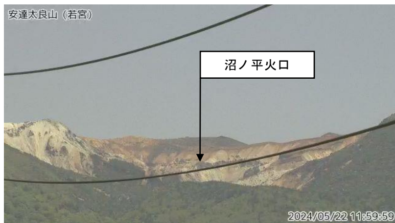
図1 安達太良山 沼ノ平火口周辺の状況（5月22日）
