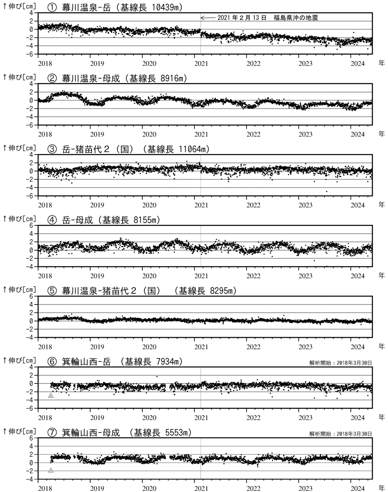
図4 安達太良山 GNSS 基線長変化図（2018年1月～2024年5月）
