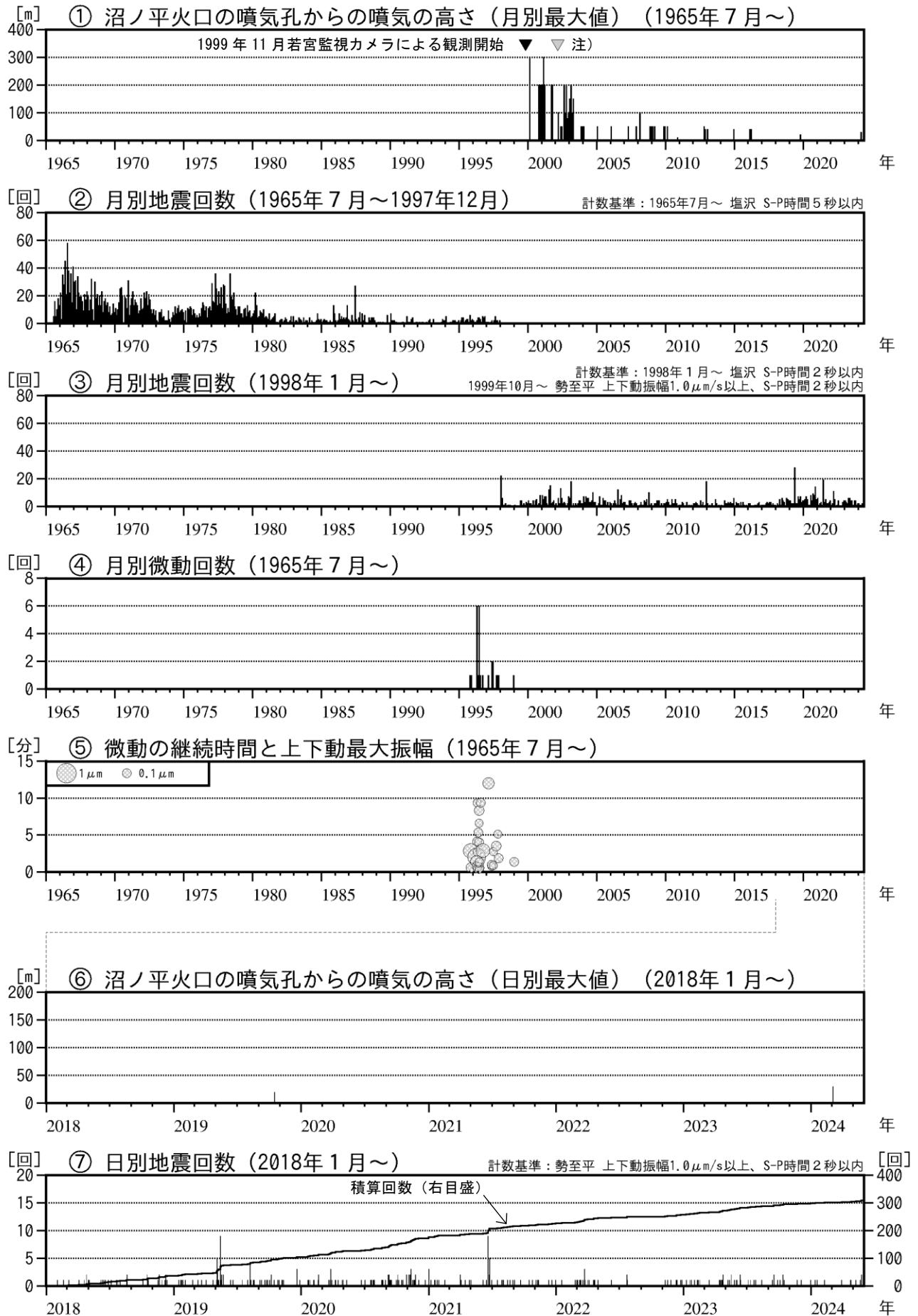
図3 安達太良山 火山活動経過図（1965年7月～2024年5月）
