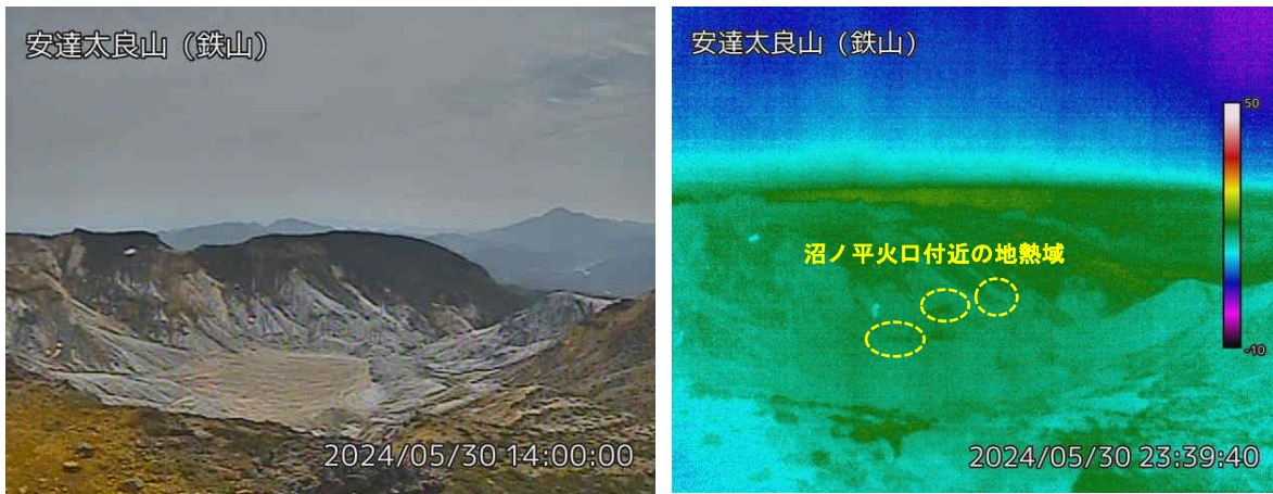
図2 安達太良山 沼ノ平火口周辺の状況と地表面温度分布の状況（5月30日）
