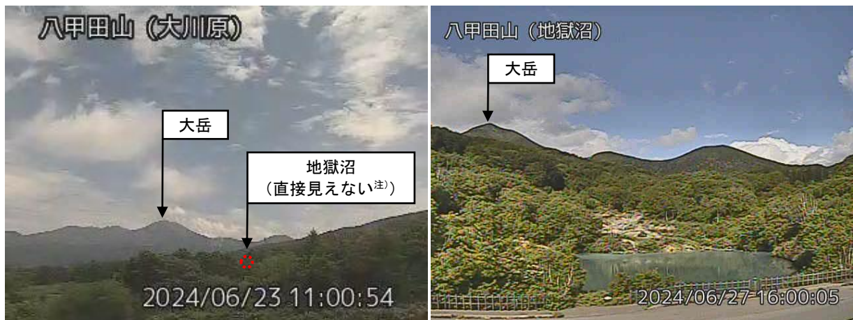
図1 八甲田山 山頂部（6月23日）及び地獄沼周辺（6月27日）の状況
