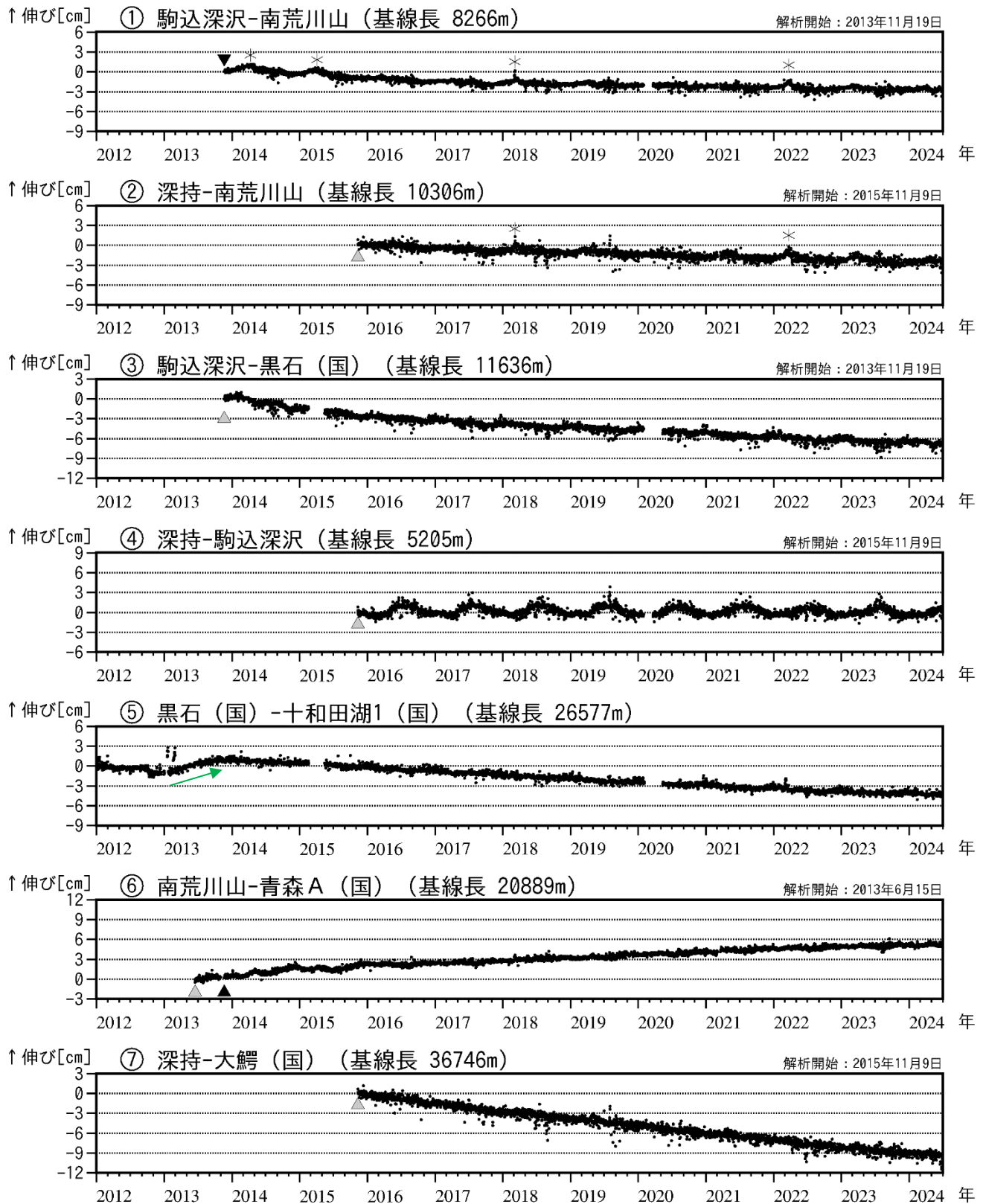
図3 八甲田山 GNSS 基線長変化図（2012年1月～2024年6月）
