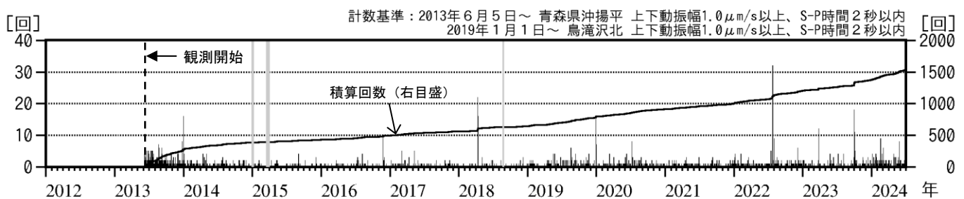
図2 八甲田山 日別地震回数（2013年6月～2024年6月）
