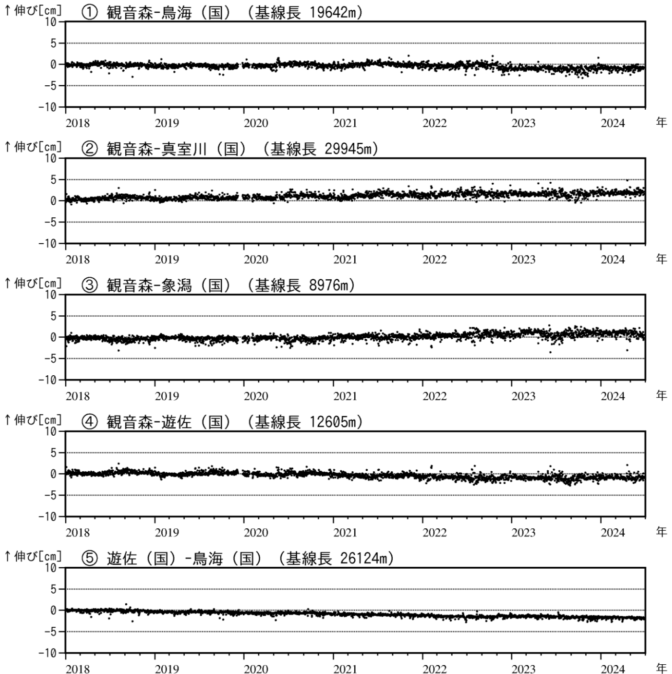
図4 鳥海山 GNSS 基線長変化図（2018年1月～2024年6月）
