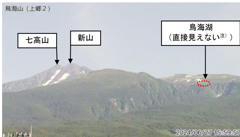
図1 鳥海山 山頂周辺の状況（6月27日）
