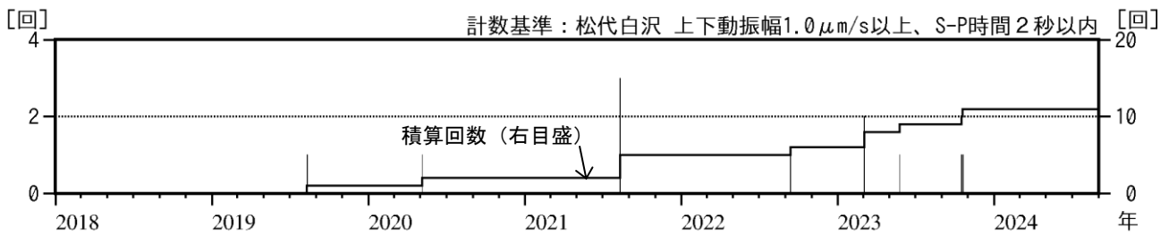
図2 岩木山 日別地震回数（2018年1月～2024年8月）
