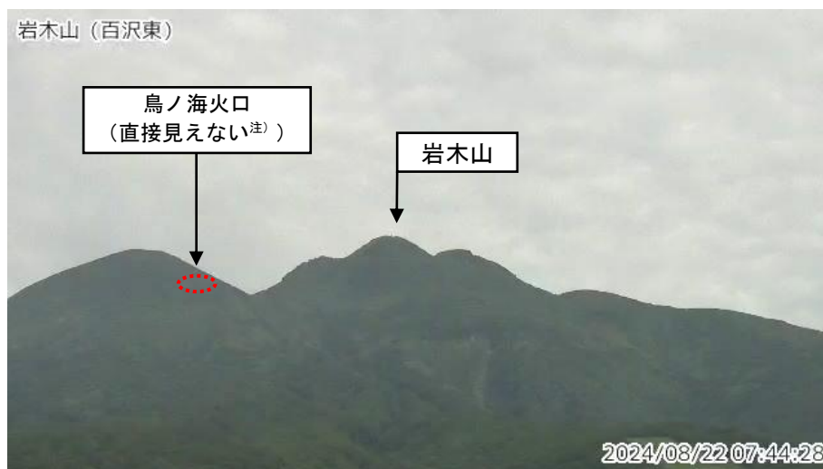
図1 岩木山 山頂部の状況（8月22日）
