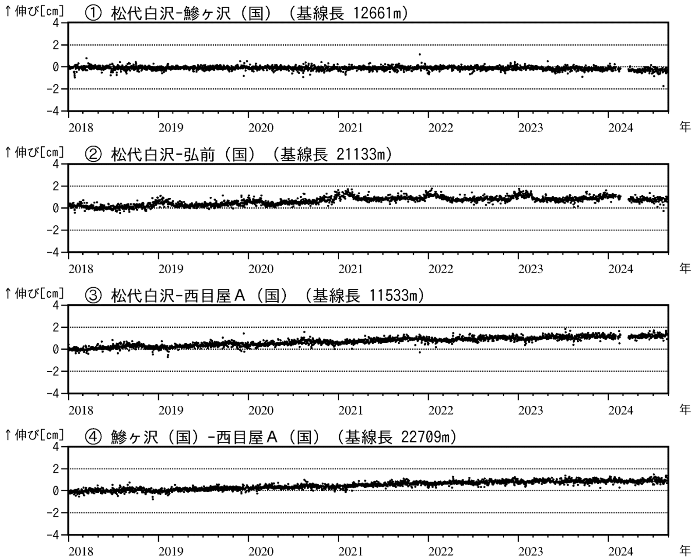
図3 岩木山 GNSS 基線長変化図（2018年1月～2024年8月）
