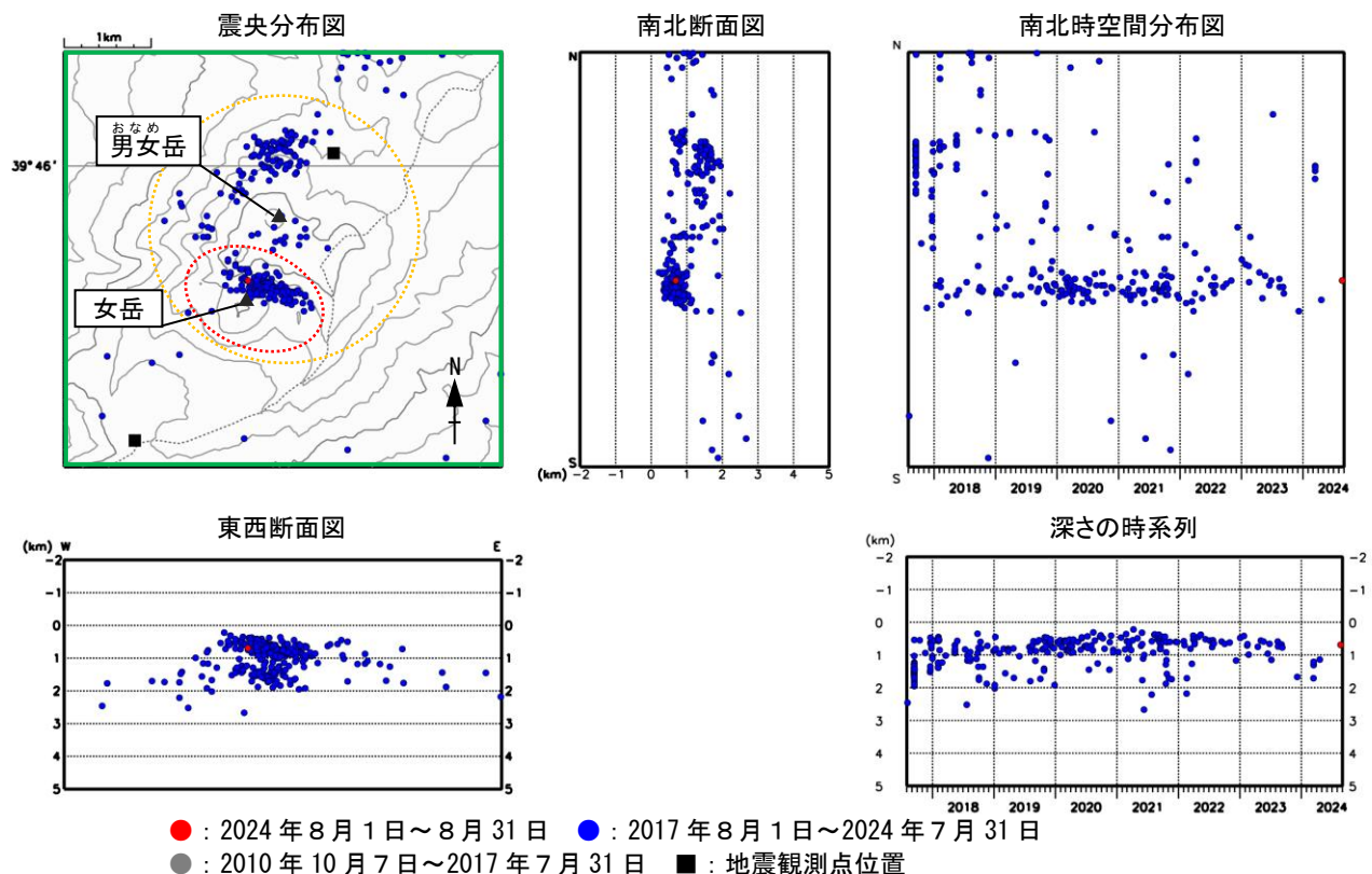
図4 秋田駒ヶ岳 地震活動（2010年10月7日～2024年8月）
