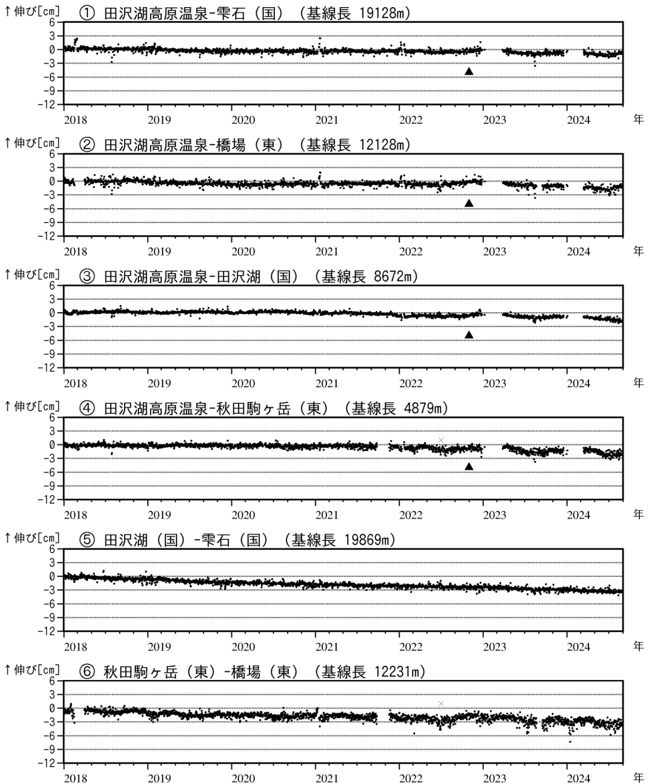
図5 秋田駒ヶ岳 GNSS 基線長変化図（2018年1月～2024年8月）
