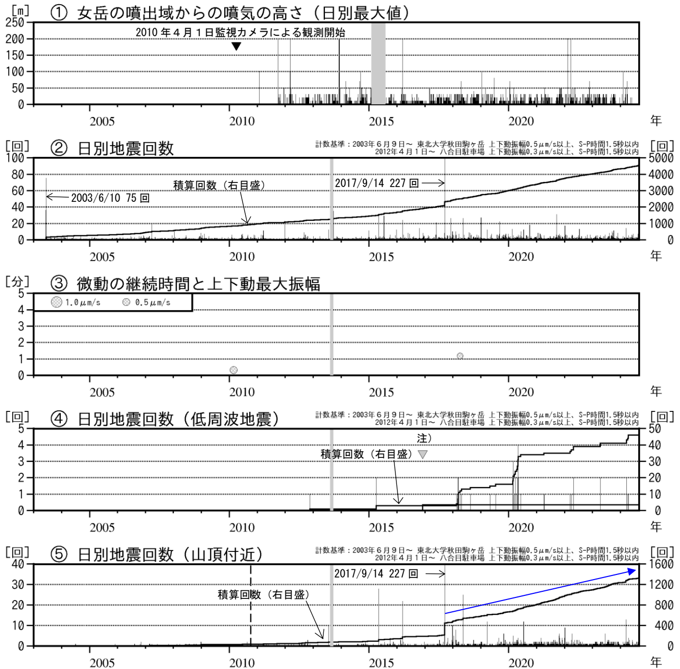
図2 秋田駒ヶ岳 火山活動経過図（2003年6月～2024年8月）
