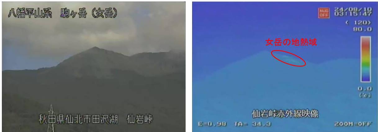
図1 秋田駒ヶ岳 女岳周辺の状況と地表面温度分布の状況（8月10日）
