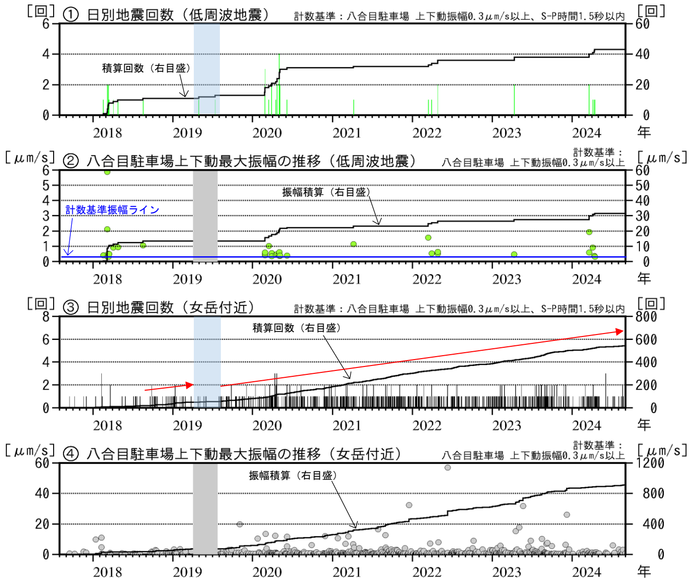
図3 秋田駒ヶ岳 低周波地震及び女岳付近の日別回数と最大振幅（2017年8月～2024年8月）
