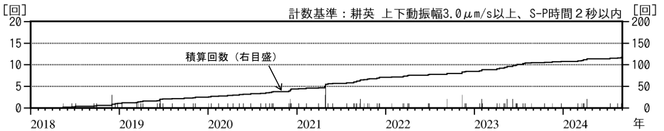
図2 栗駒山 日別地震回数（2018年1月～2024年8月）
