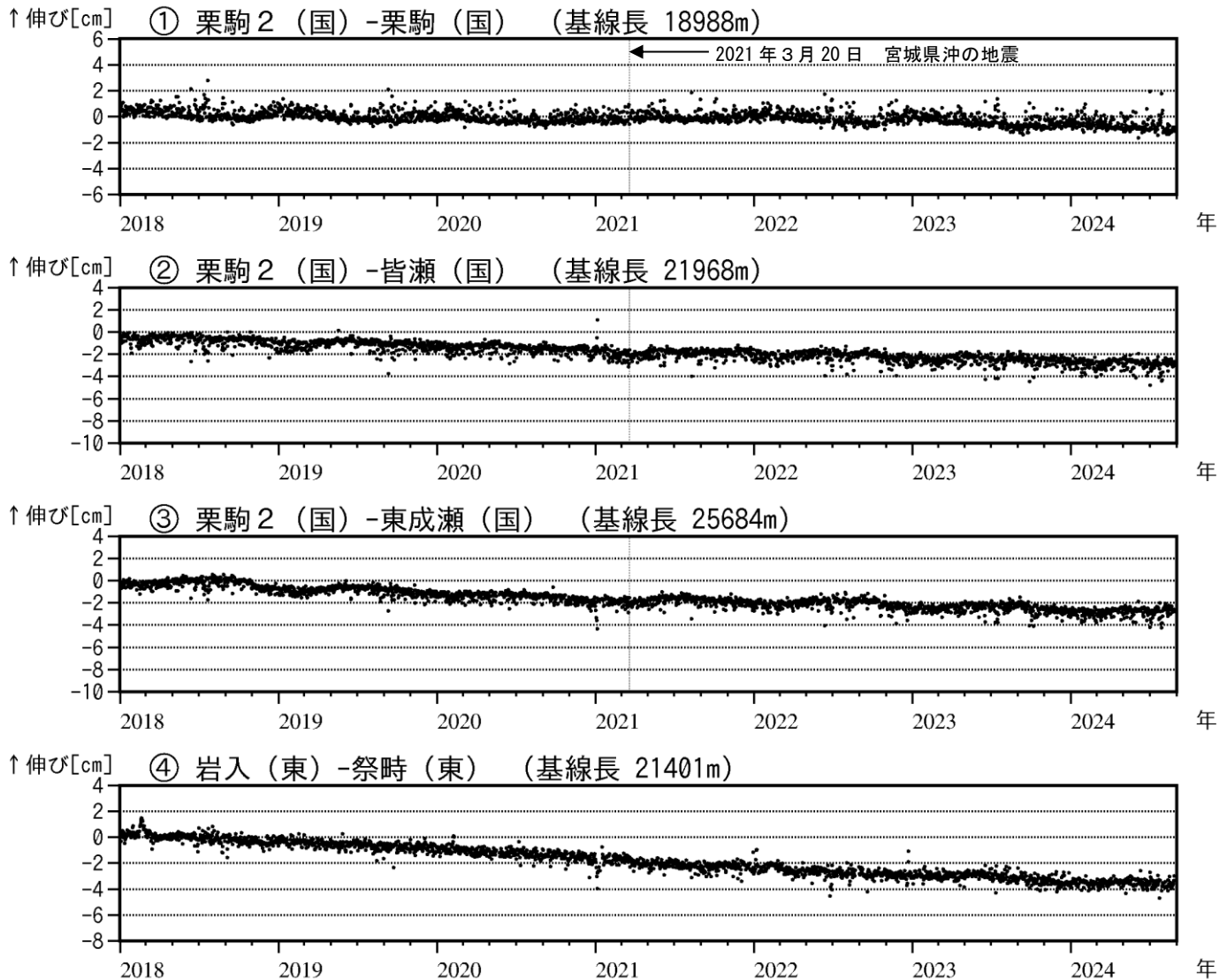
図3 栗駒山 GNSS 基線長変化図（2018年1月～2024年8月）
