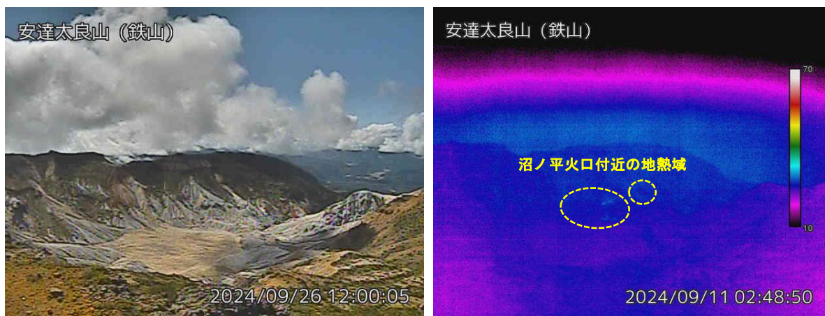
図2 安達太良山 沼ノ平火口周辺の状況（9月26日）と地表面温度分布の状況（9月11日） ・鉄山監視カメラ（沼ノ平火口の北東約700m）の映像です。
