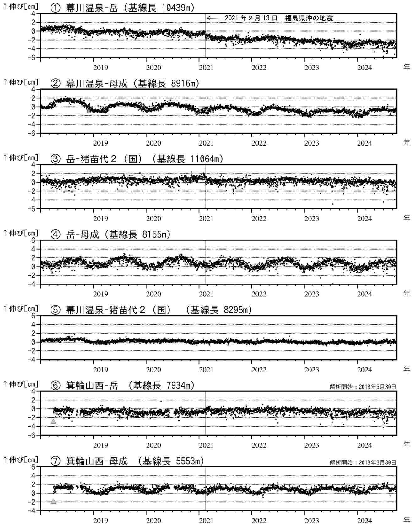
図4 安達太良山 GNSS 基線長変化図（2018年1月～2024年9月）
