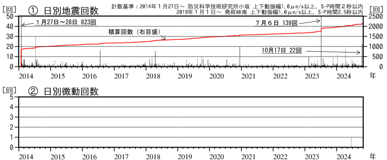
図2 十和田 活動経過図（2014年1月～2024年10月）
