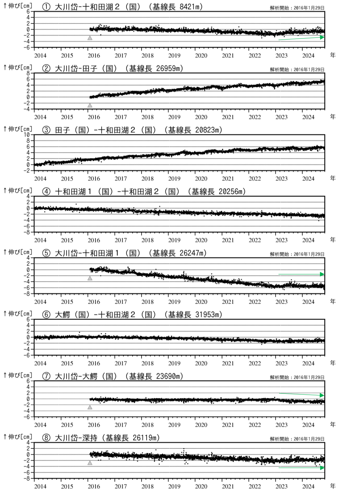
図3 十和田 GNSS 基線長変化図 (2014年1月～2024年10月)
