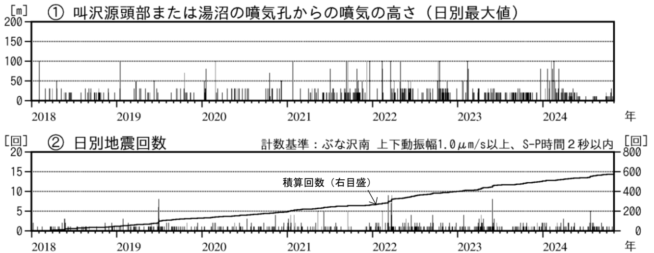
図3 秋田焼山 火山活動経過図（2018年1月～2024年10月）
