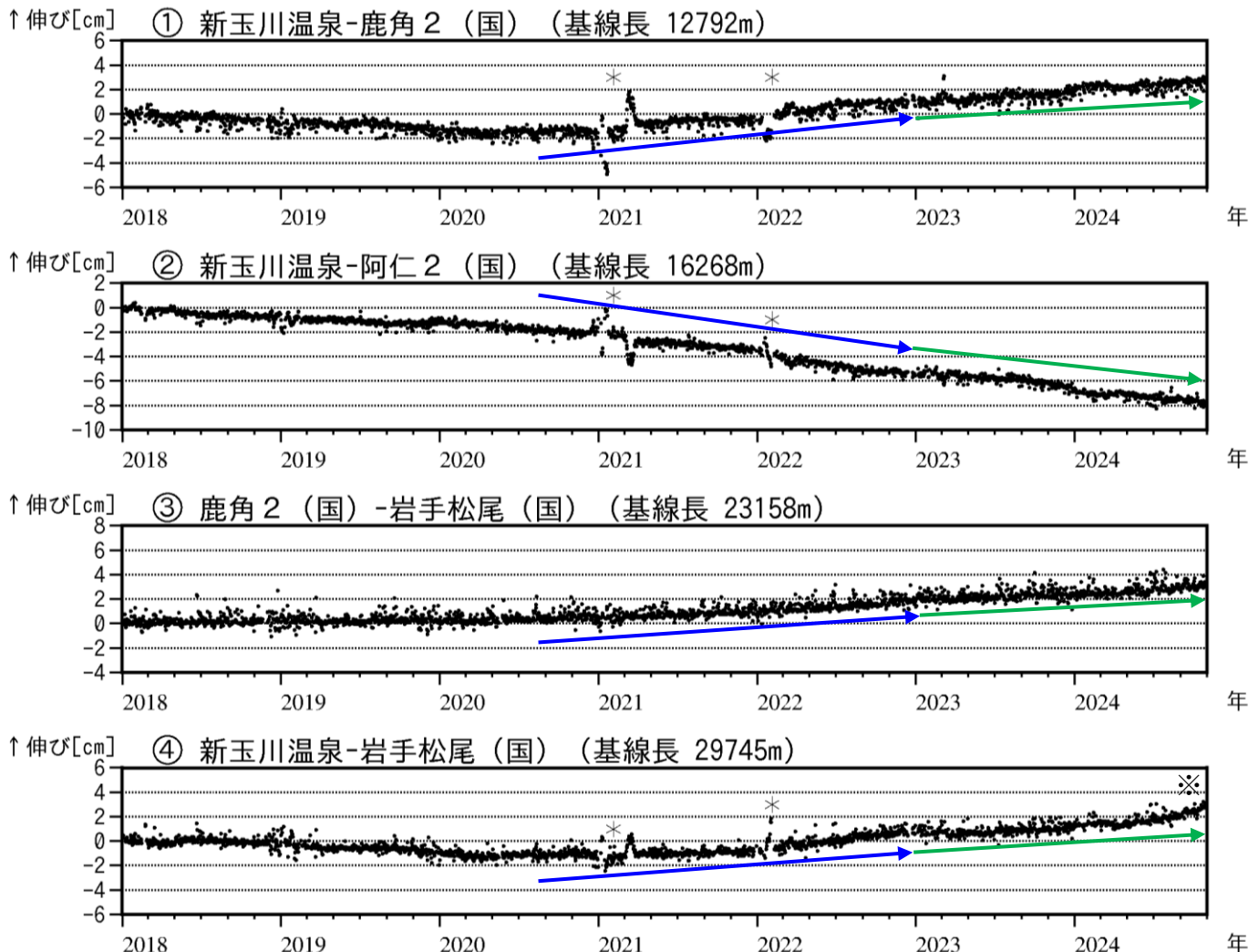
図4 秋田焼山 GNSS 基線長変化図（2018年1月～2024年10月）
