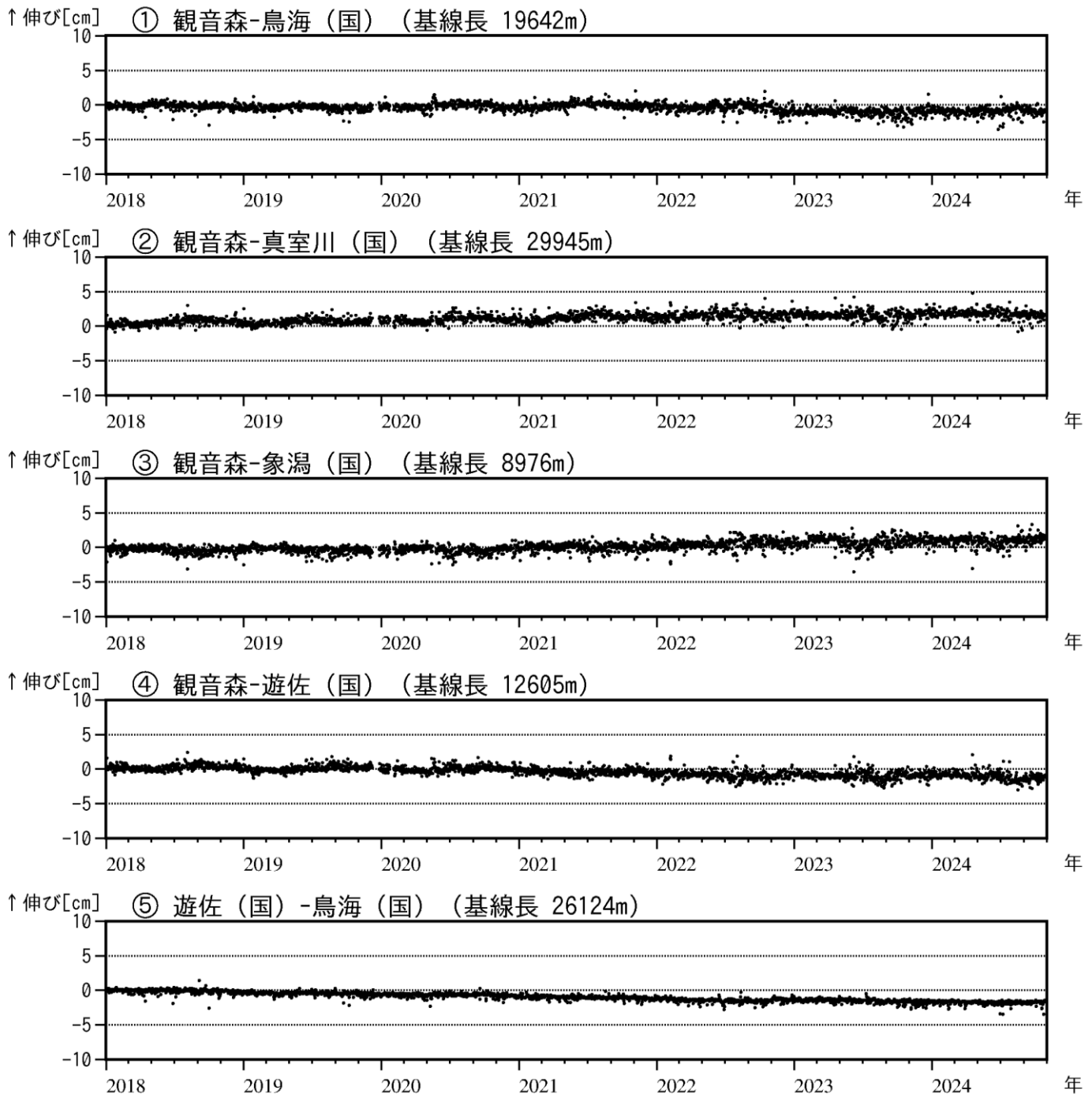
図4 鳥海山 GNSS 基線長変化図（2018年1月～2024年10月）
