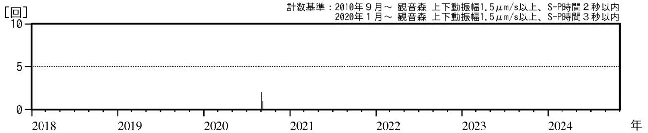
図3 鳥海山 火山性地震の日別回数（2018年1月～2024年10月）
