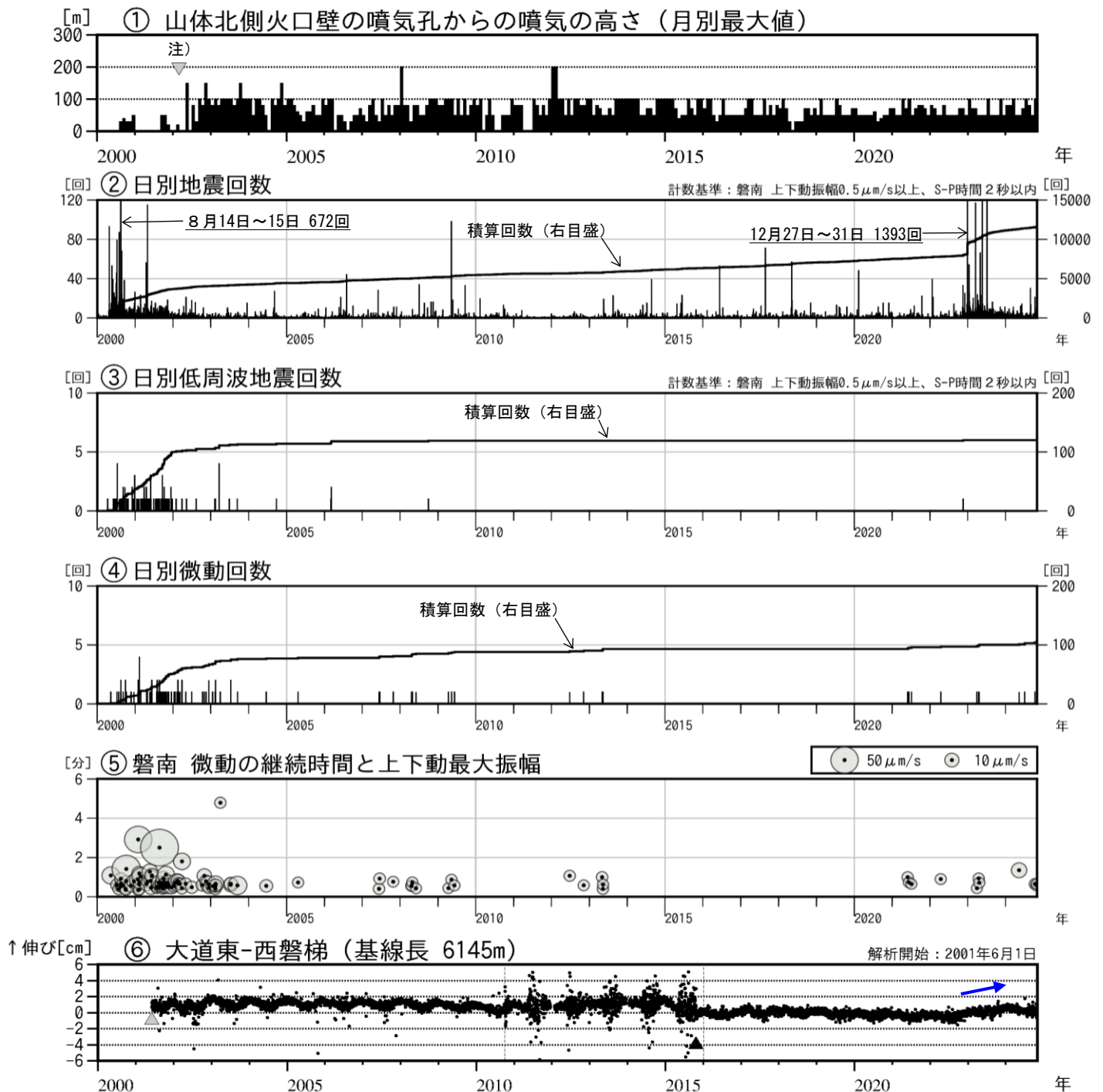
図4 磐梯山 火山活動経過図（2000年1月～2024年10月）
