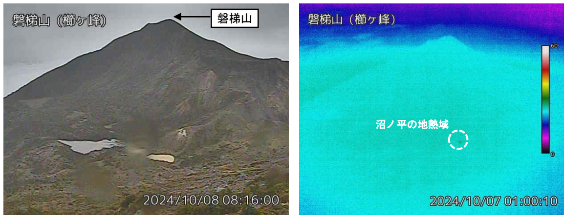
図2 磐梯山 沼ノ平周辺の状況（10月8日）と地表面温度分布（10月7日）
