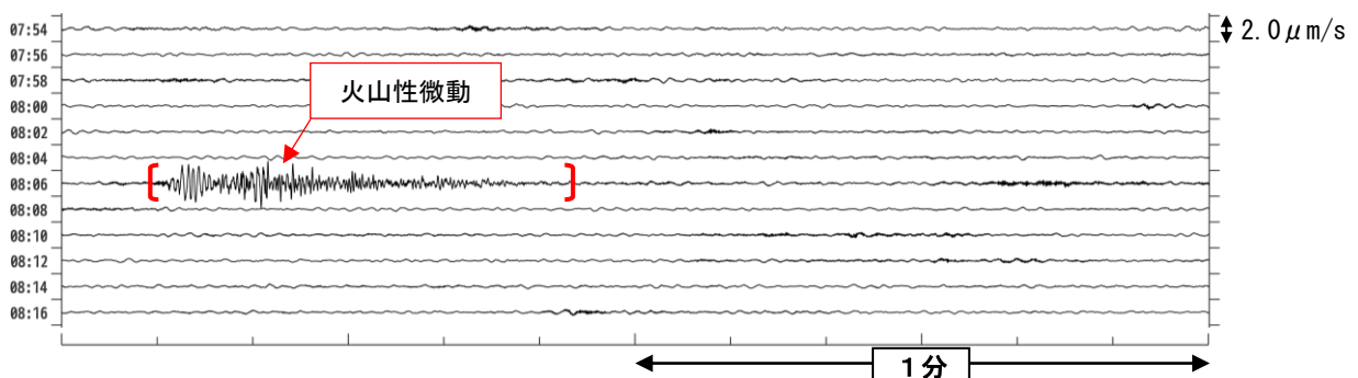
図3 磐梯山 裏磐梯高原観測点（上下成分）での火山性微動の発生状況（2024年10月27日07時54分～08時18分）
