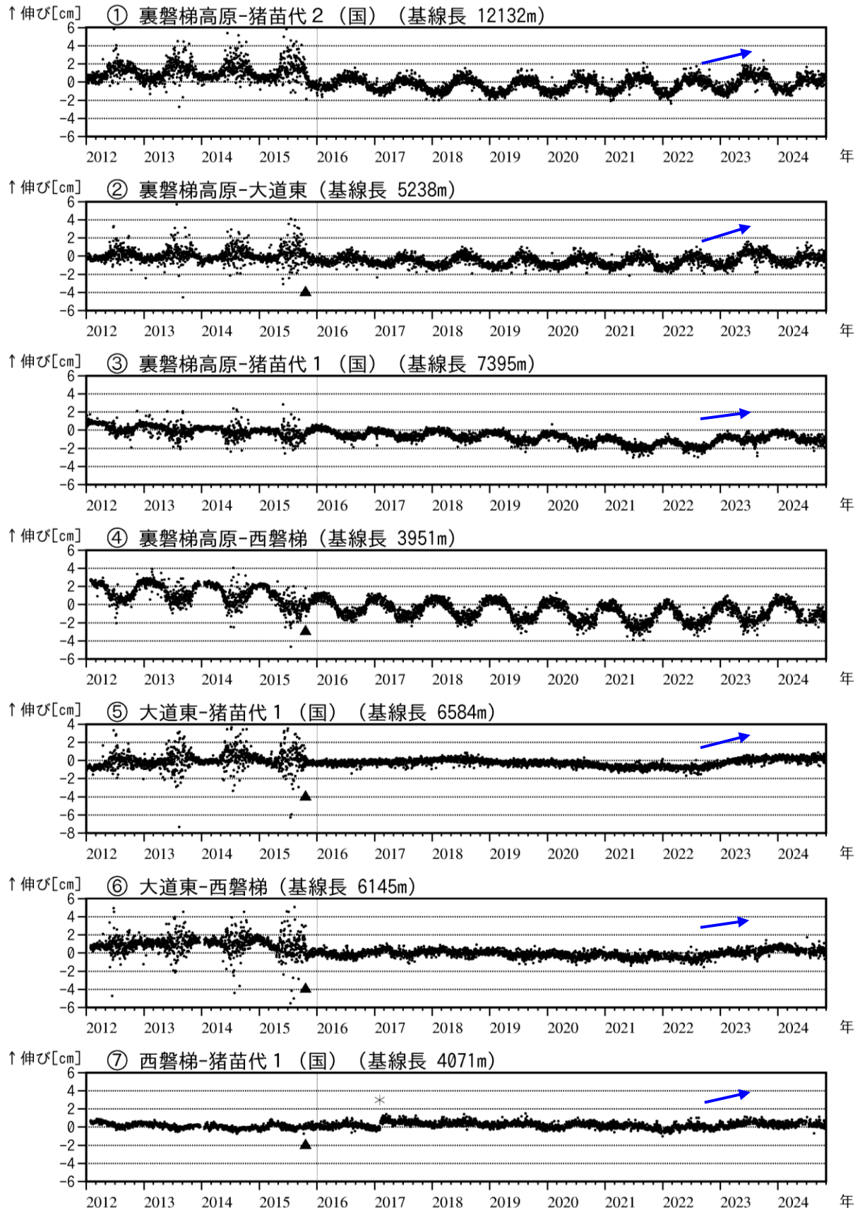
図7 磐梯山 GNSS基線長変化図（2012年1月～2024年10月）
