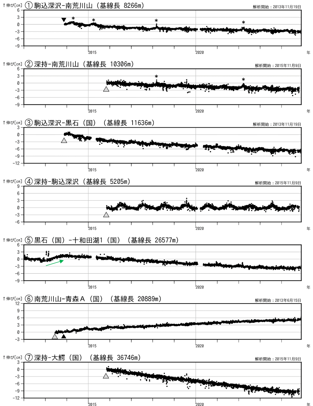
図3 八甲田山 GNSS 基線長変化図（2012年1月～2024年11月）
