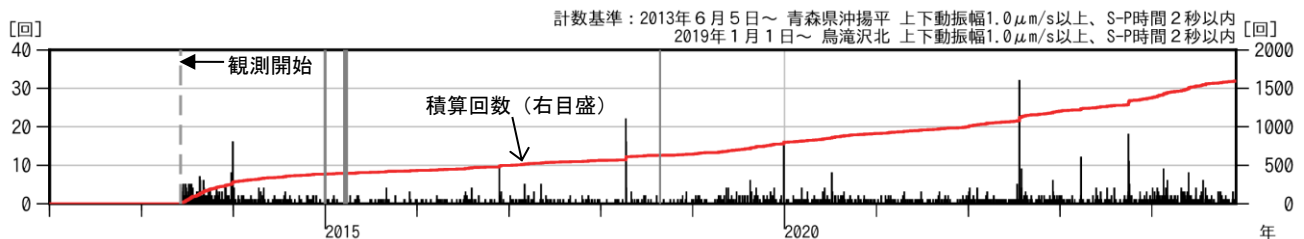
図2 八甲田山 日別地震回数（2013年6月～2024年11月）
