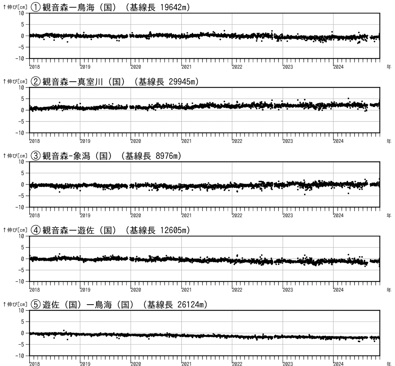
図4 鳥海山 GNSS 基線長変化図（2018年1月～2024年11月）
