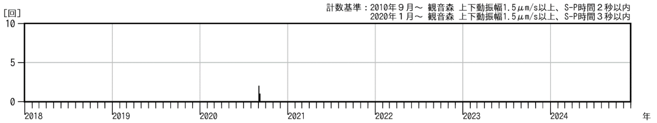
図3 鳥海山 火山性地震の日別回数（2018年1月～2024年11月）
