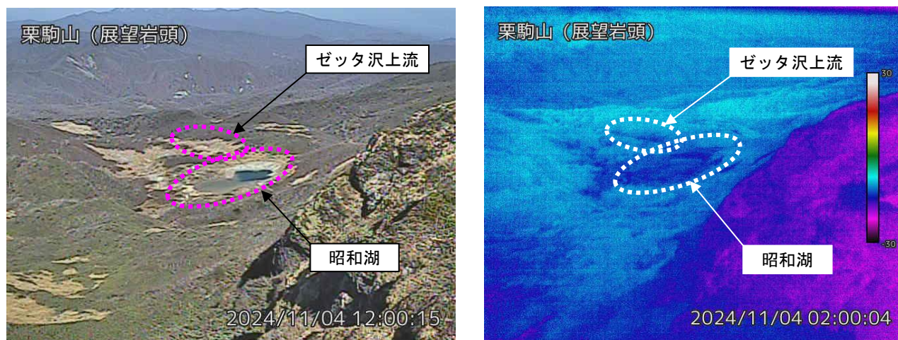
図2 栗駒山 昭和湖及びゼッタ沢上流周辺の状況と地表面温度分布（11月4日）
