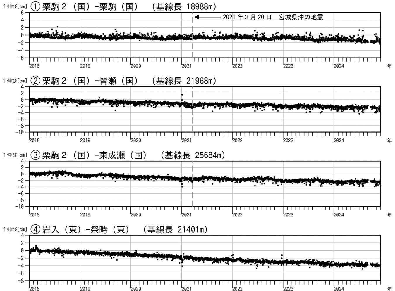
図4 栗駒山 GNSS 基線長変化図（2018年1月～2024年11月）
