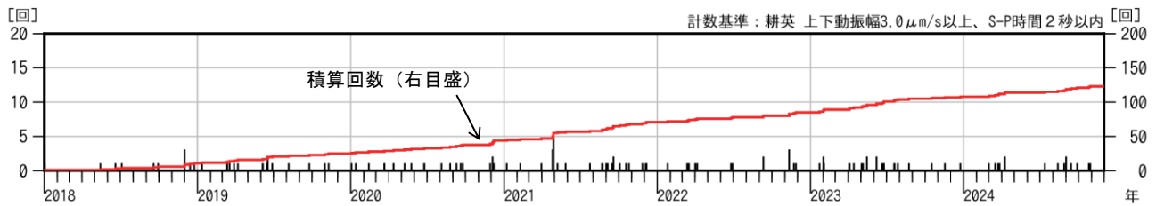
図3 栗駒山 日別地震回数（2018年1月～2024年11月）
