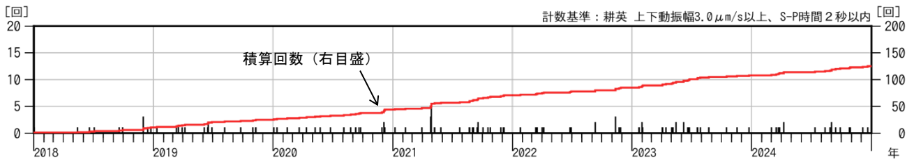
図2 栗駒山 日別地震回数（2018年1月～2024年12月）
