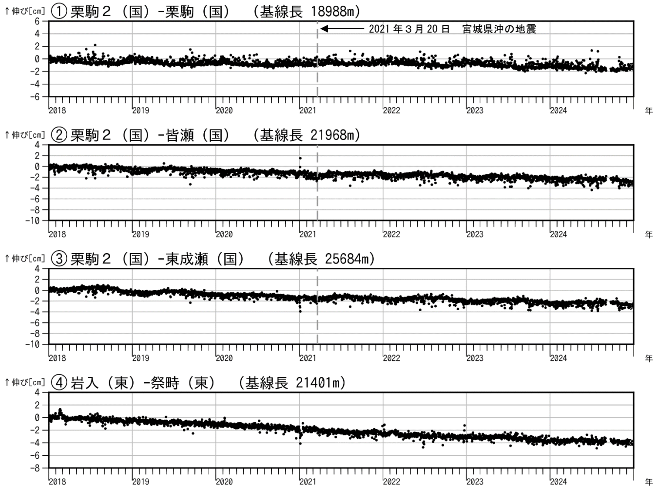
図3 栗駒山 GNSS 基線長変化図（2018年1月～2024年12月）
