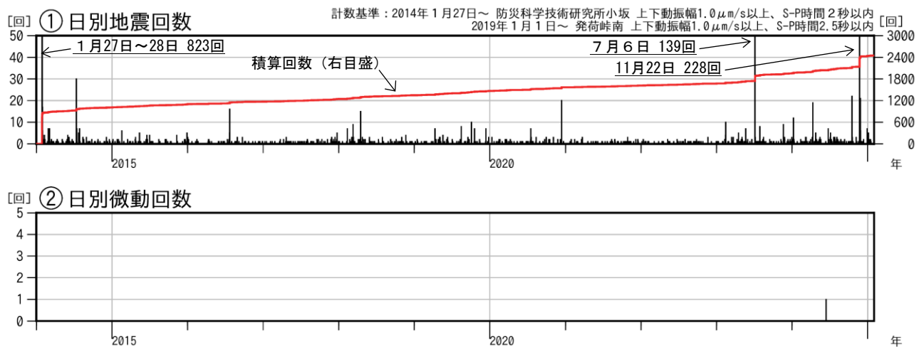
図2 十和田 活動経過図（2014年1月～2025年1月）
