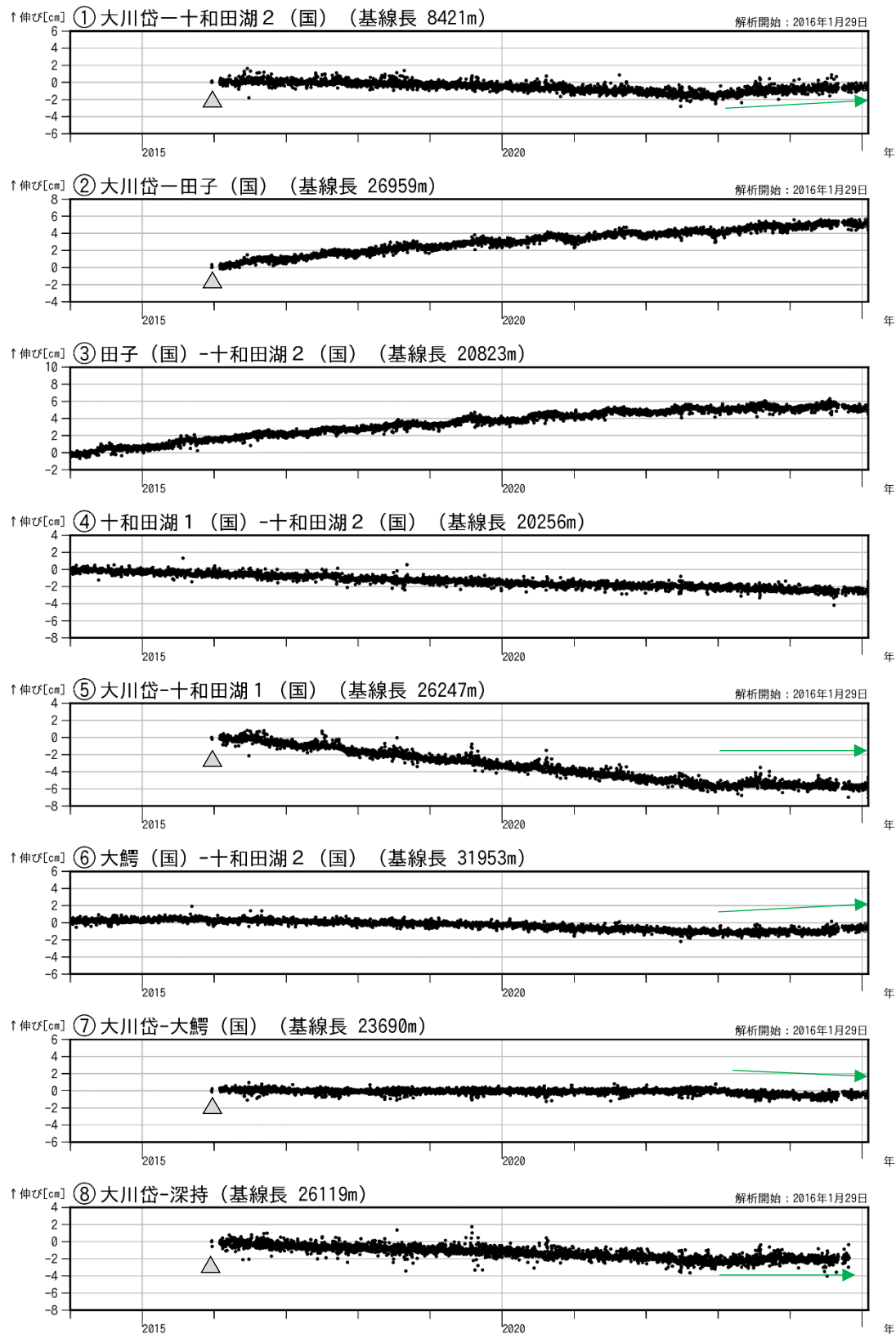
図3 十和田 GNSS 基線長変化図（2014年1月～2025年1月）
