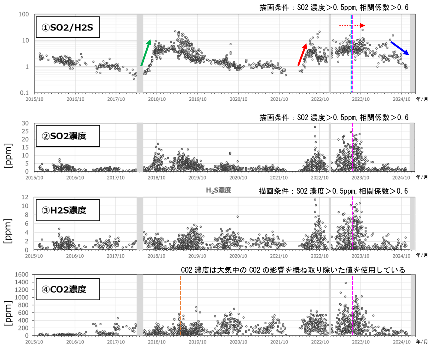
図6 吾妻山 火山ガス観測装置による観測（2015年11月～2025年1月）
