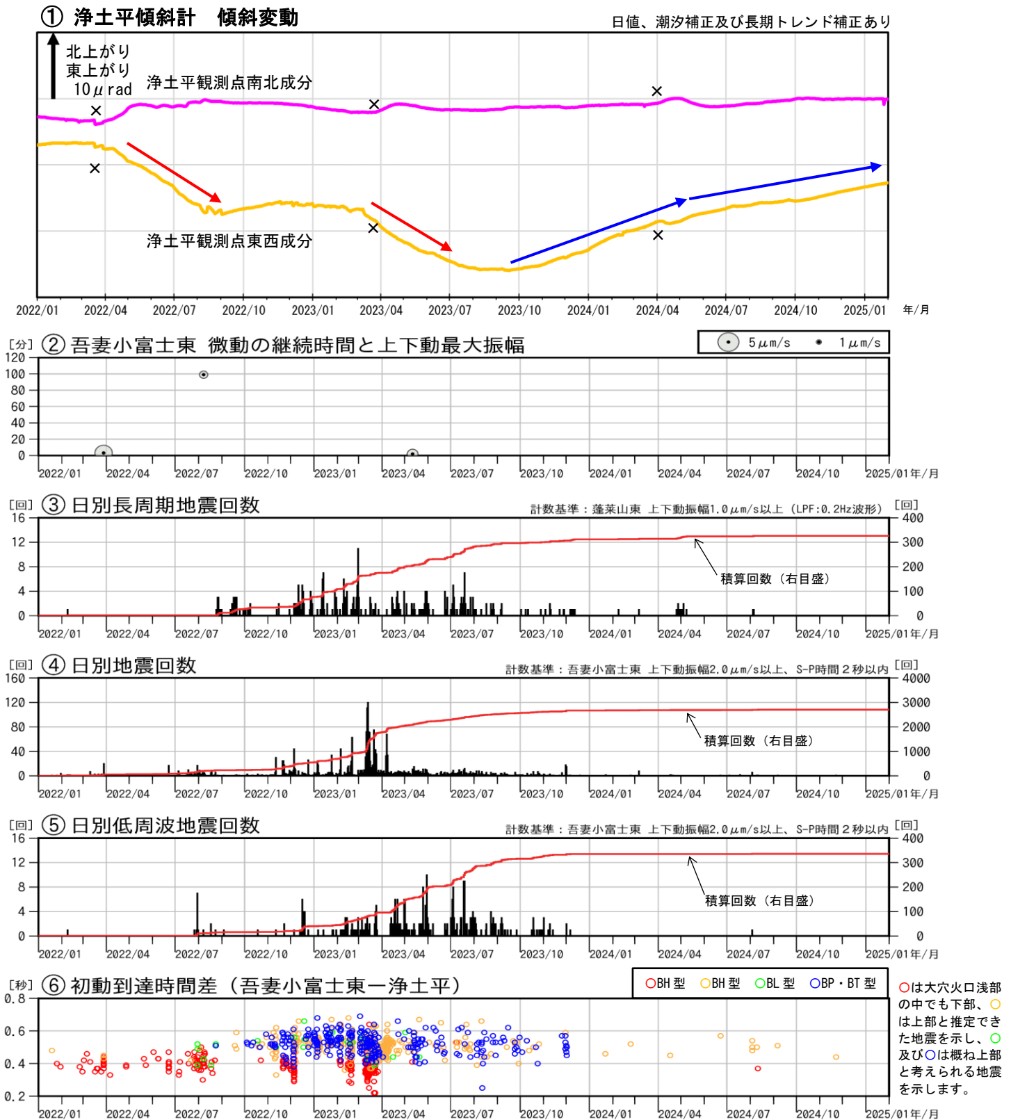
図3 吾妻山 火山活動経過図（2022年1月～2025年1月）
