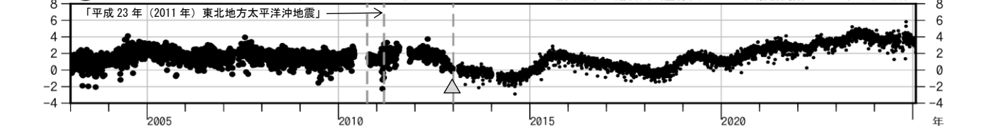
図2 吾妻山 中期的な火山活動の経過（2003年1月～2025年1月）
