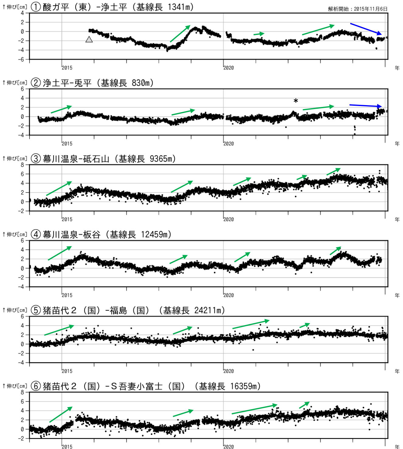
図4 吾妻山 吾妻山浅部・深部の地殻変動（2014年1月～2025年1月）
