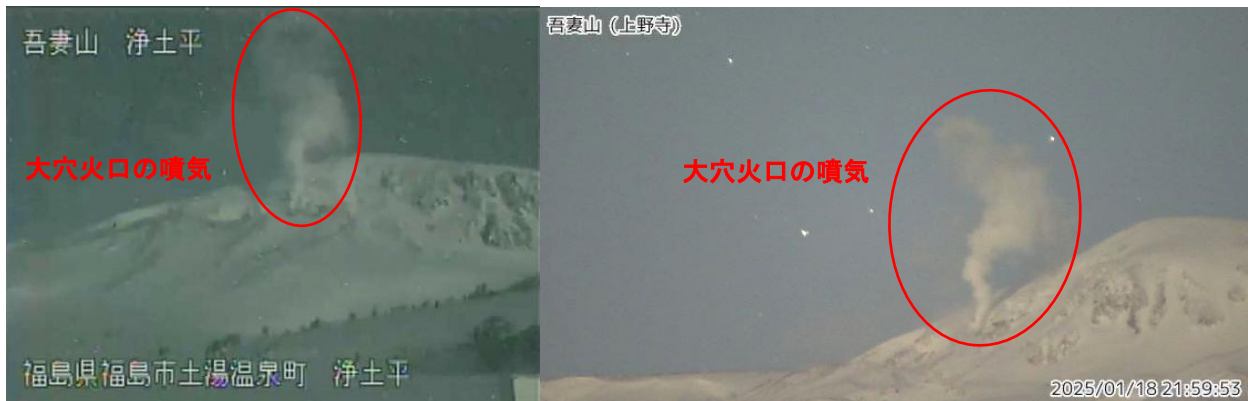
図1 吾妻山 大穴火口周辺の噴気の状態（1月18日）
