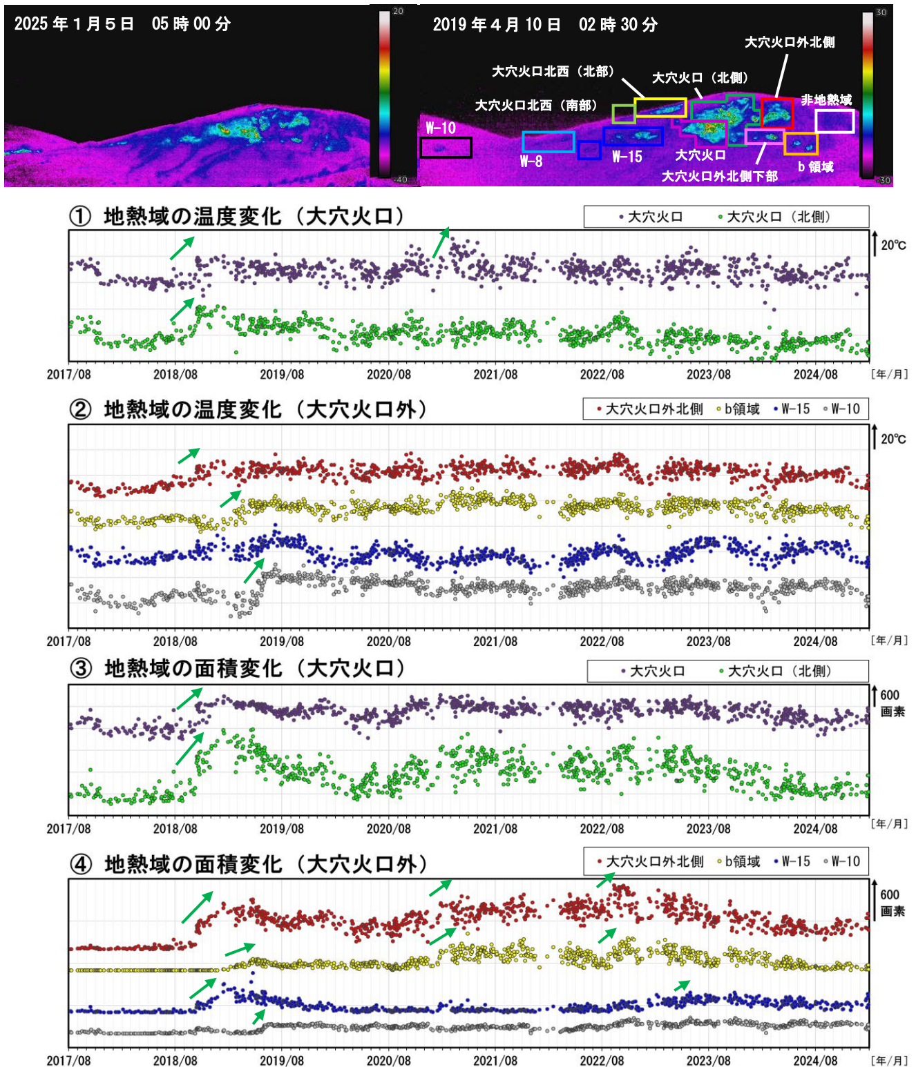
図5 吾妻山 監視カメラによる大穴火口周辺の地熱域の経過（2017 年 8 月～2025 年 1 月）
