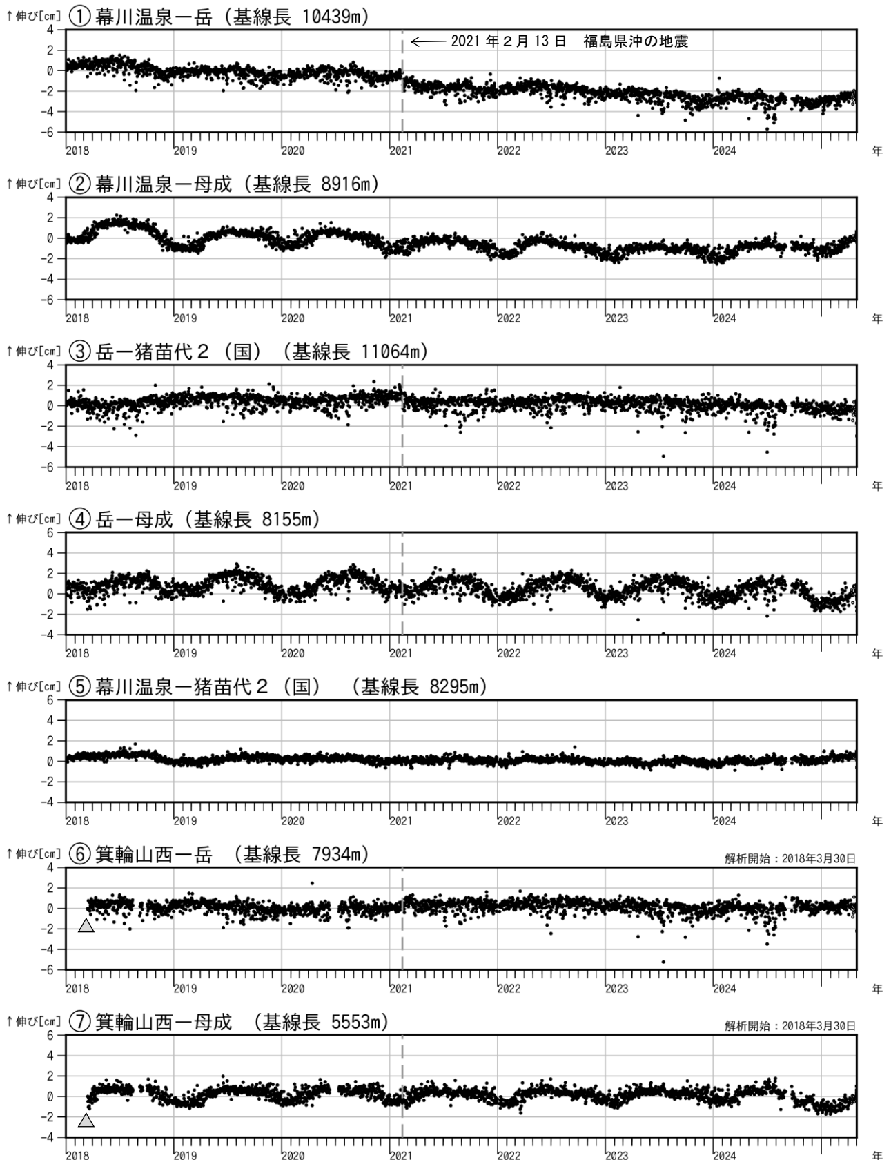
図4 安達太良山 GNSS 基線長変化図（2018年1月～2025年4月）
