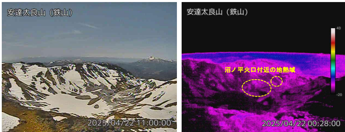
図2 安達太良山 沼ノ平火口周辺の状況と地表面温度分布の状況（4月22日） ・鉄山監視カメラ（沼ノ平火口の北東約700m）の映像です。
