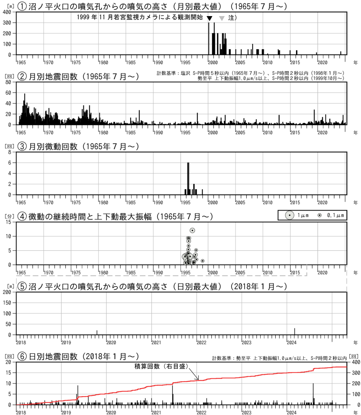
図3 安達太良山 火山活動経過図（1965年7月～2025年4月）
