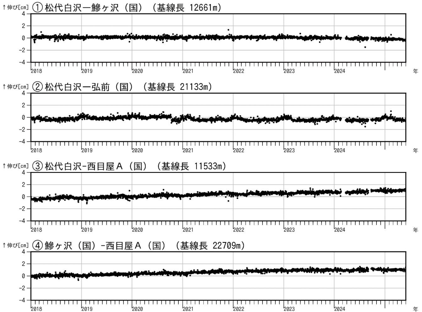
図3 岩木山 GNSS 基線長変化図（2018年1月～2025年5月）
