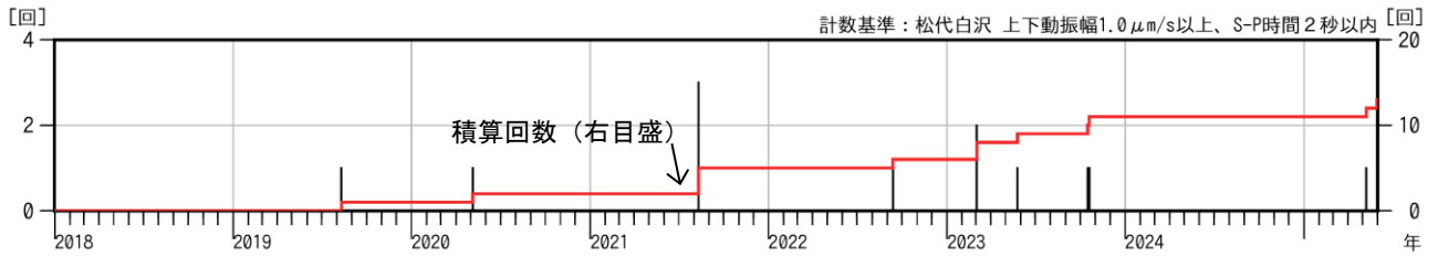
図2 岩木山 日別地震回数（2018年1月～2025年5月）
