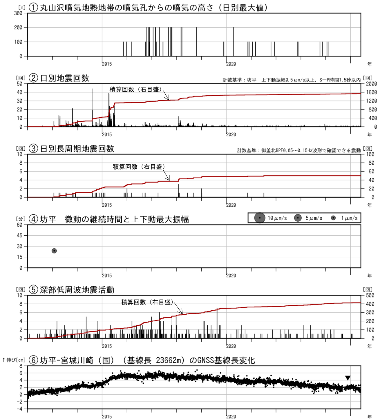
図2 蔵王山 火山活動経過図（2012年1月～2025年5月）
