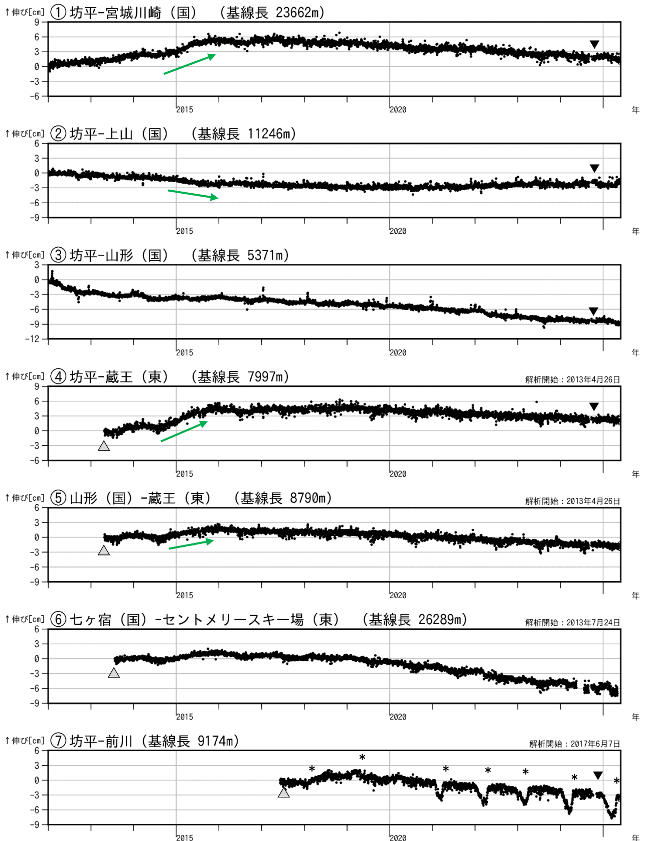
図3 蔵王山 GNSS 基線長変化図 (2012 年 1 月～2025 年 5 月)
