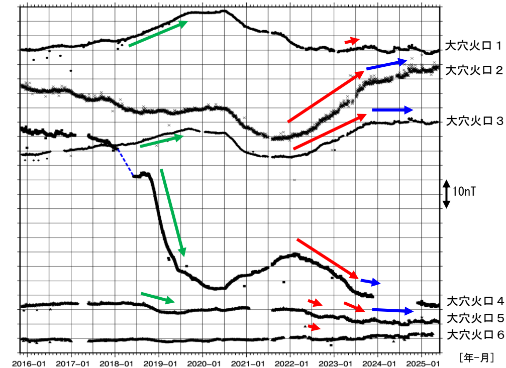
図9 吾妻山 全磁力連続観測点の全磁力値変化（2015 年 11 月～2025 年 5 月）
