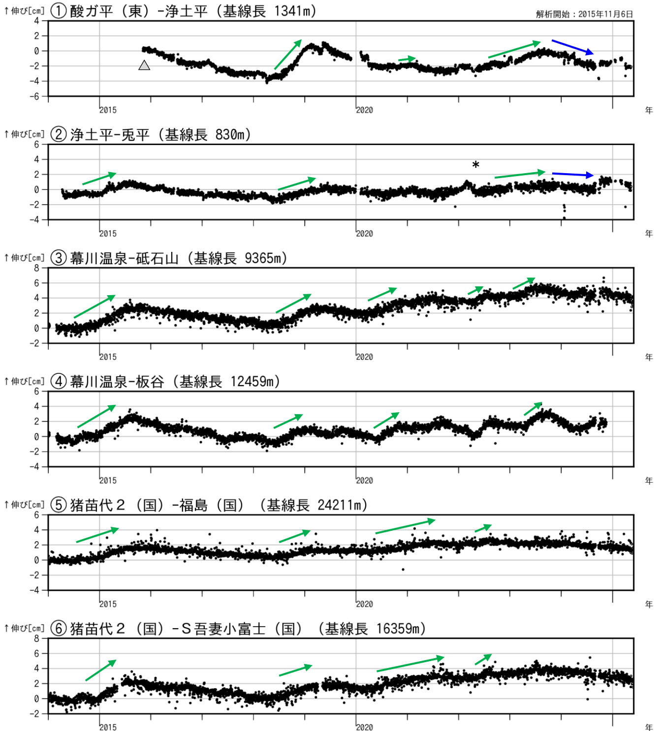
図4 吾妻山 吾妻山浅部・深部の地殻変動（2014年1月～2025年5月）
