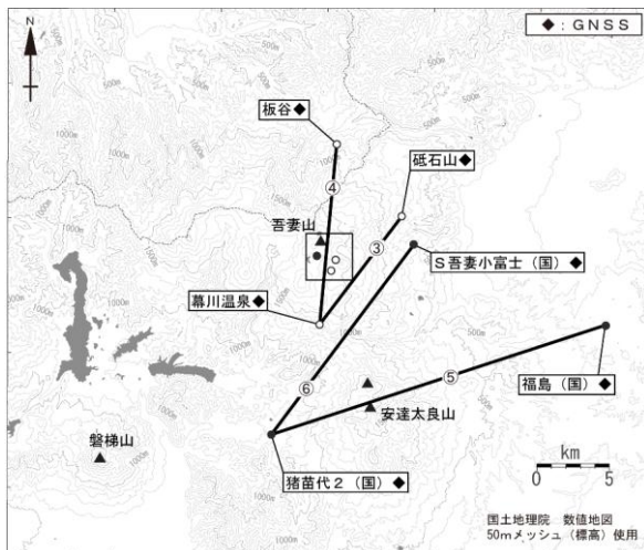
図 12 吾妻山 GNSS 観測基線図
