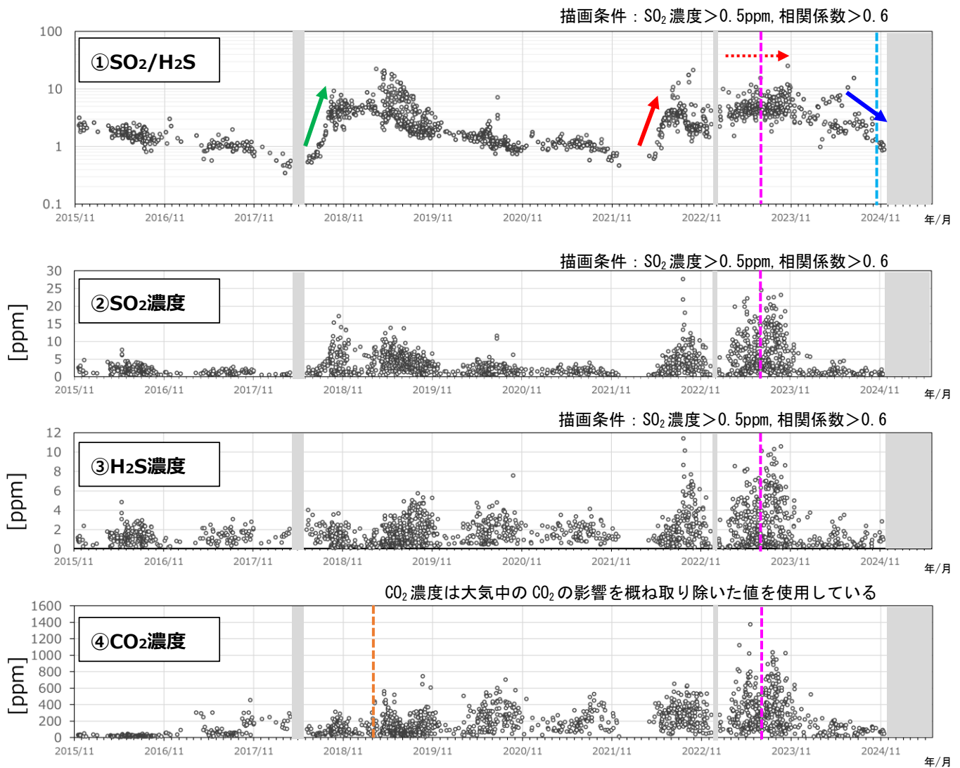
図8 吾妻山 火山ガス観測装置による観測（2015年11月～2025年5月）
