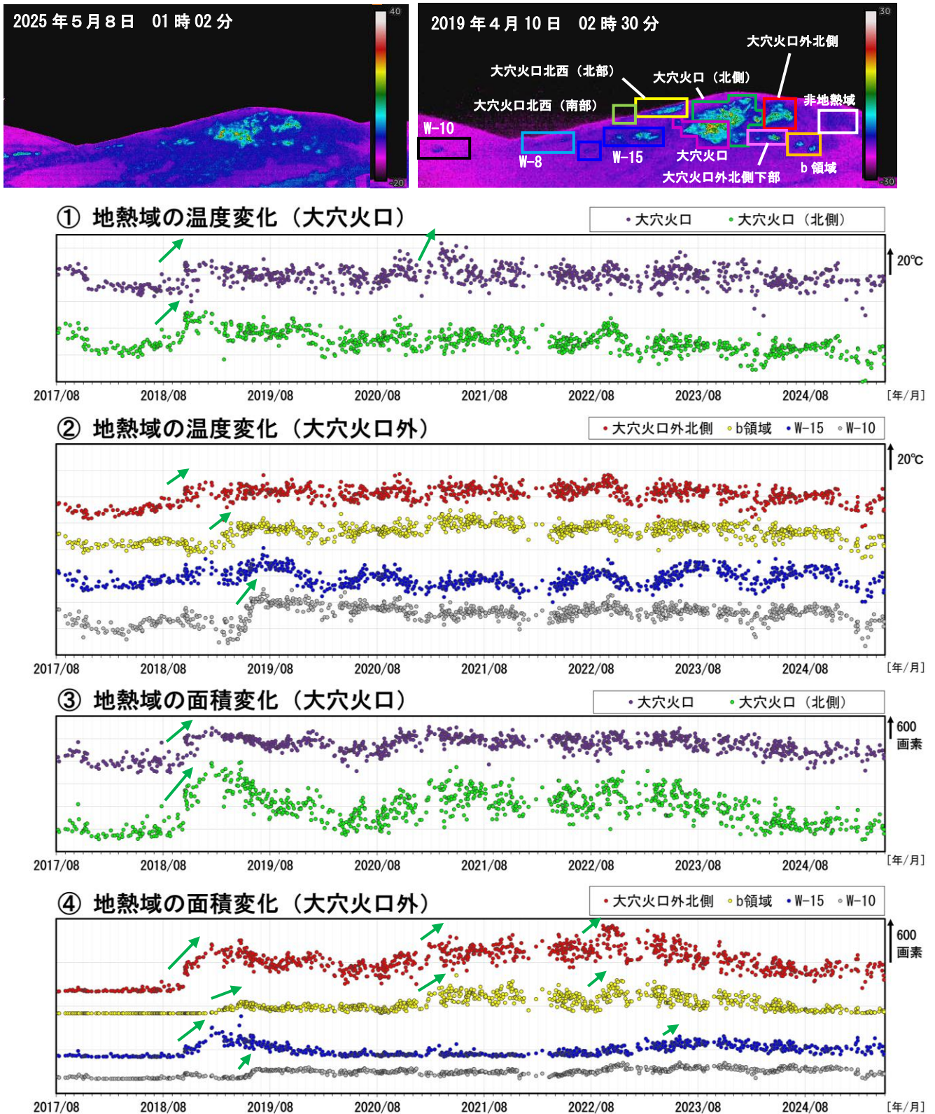
図5 吾妻山 監視カメラによる大穴火口周辺の地熱域の経過（2017 年 8 月～2025 年 5 月）
