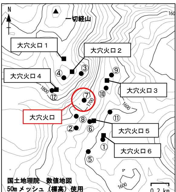
図 13 吾妻山 全磁力観測点配置図
