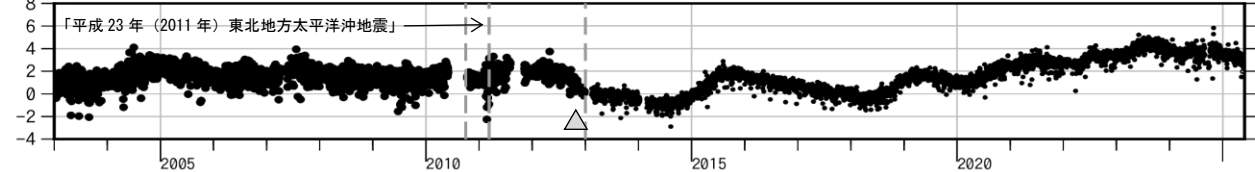
図2 吾妻山 中期的な火山活動の経過（2003年1月～2025年5月）
