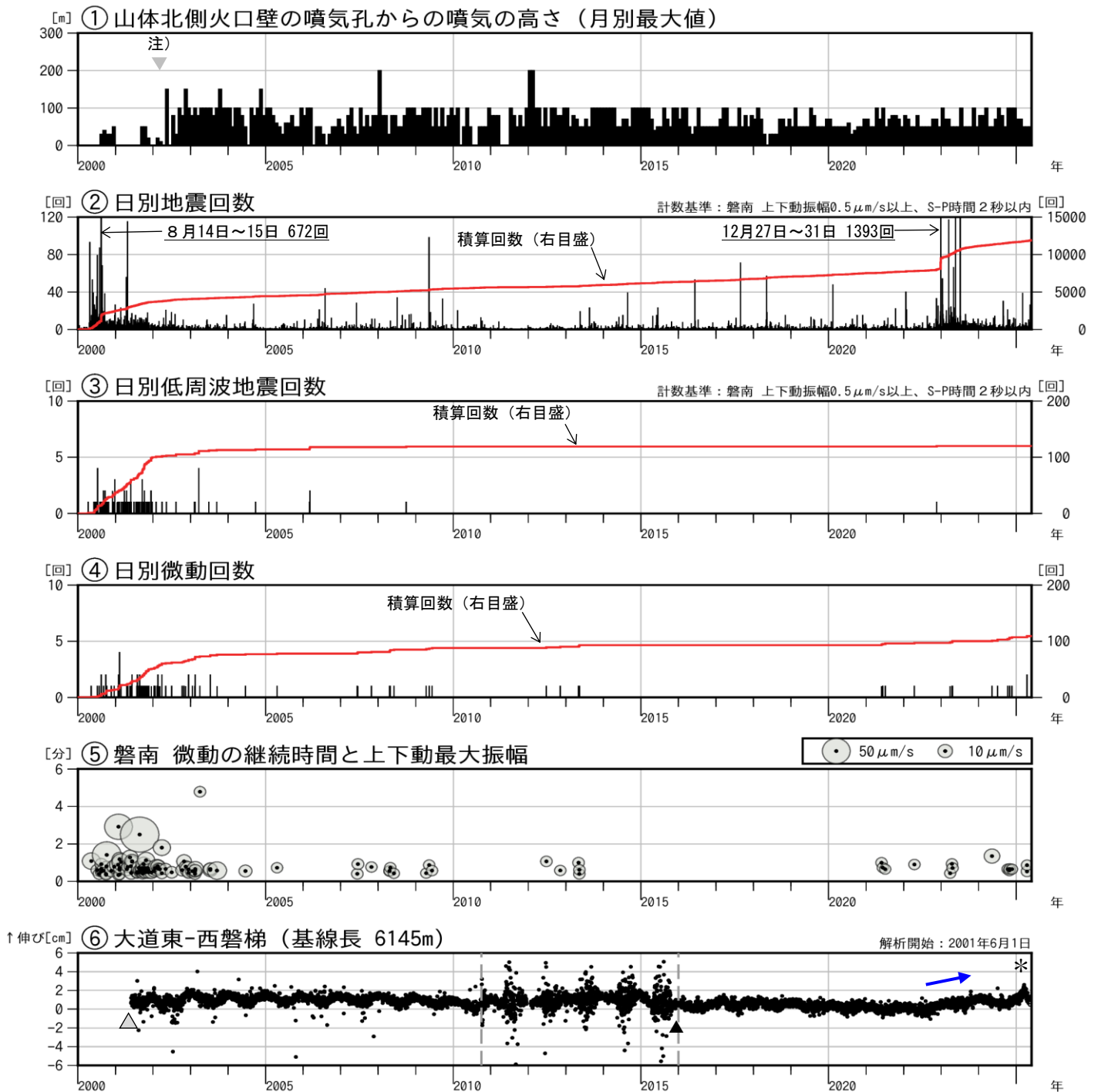
図 7 磐梯山 火山活動経過図（2000 年 1 月～2025 年 5 月）
