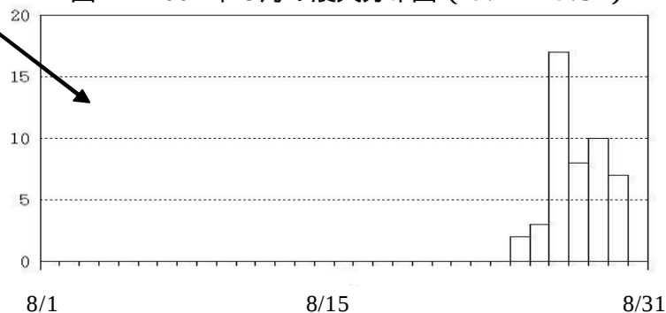
図 2 北西外輪周辺（図 1 □ 部）の地震日別回数
