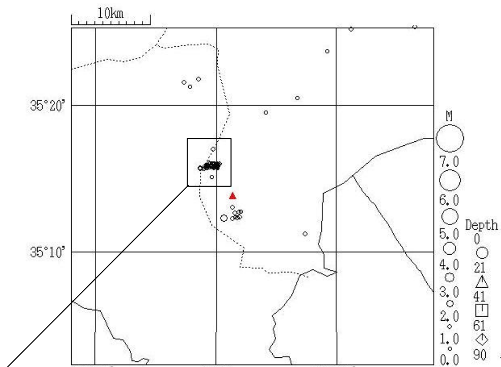
図 1 2002 年 8 月の震央分布図（8/1～8/31）
