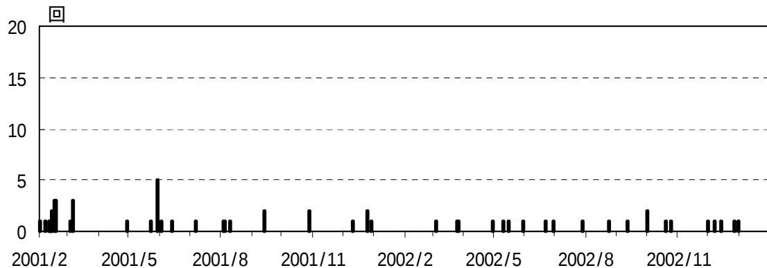
図1 富士山 高周波地震日別回数(2001年2月1日～2003年1月31日)
