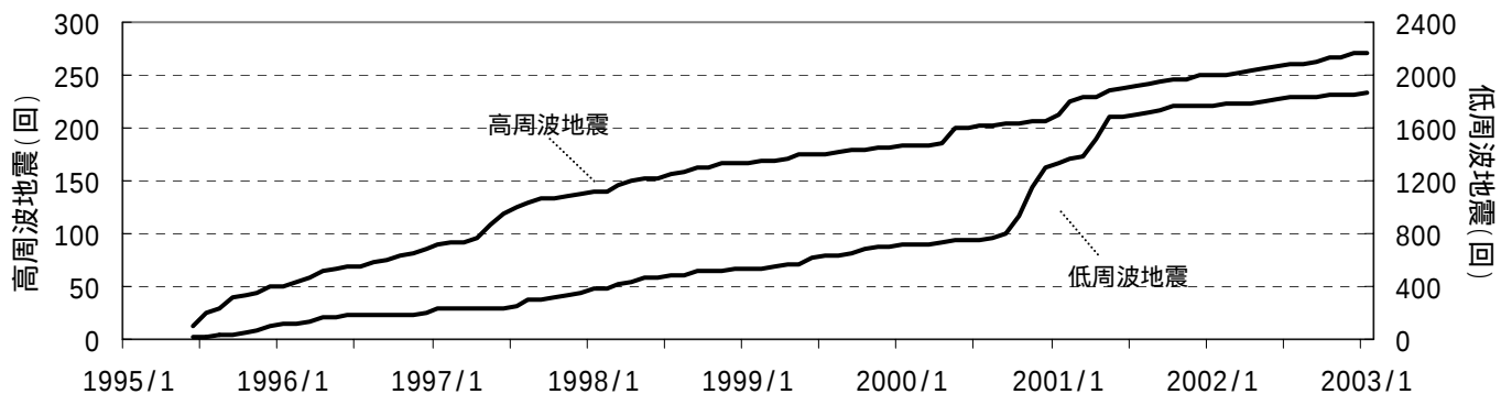
図5 富士山 地震積算回数(1995年6月～2003年1月)
