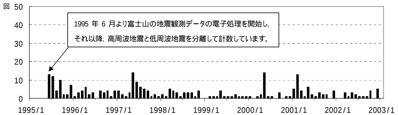
図3 富士山 高周波地震月別回数(1995年6月～2003年1月)
