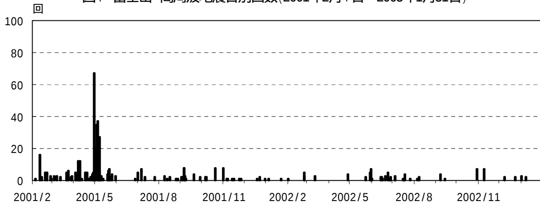
図2 富士山 低周波地震日別回数(2001年2月1日～2003年1月31日)
