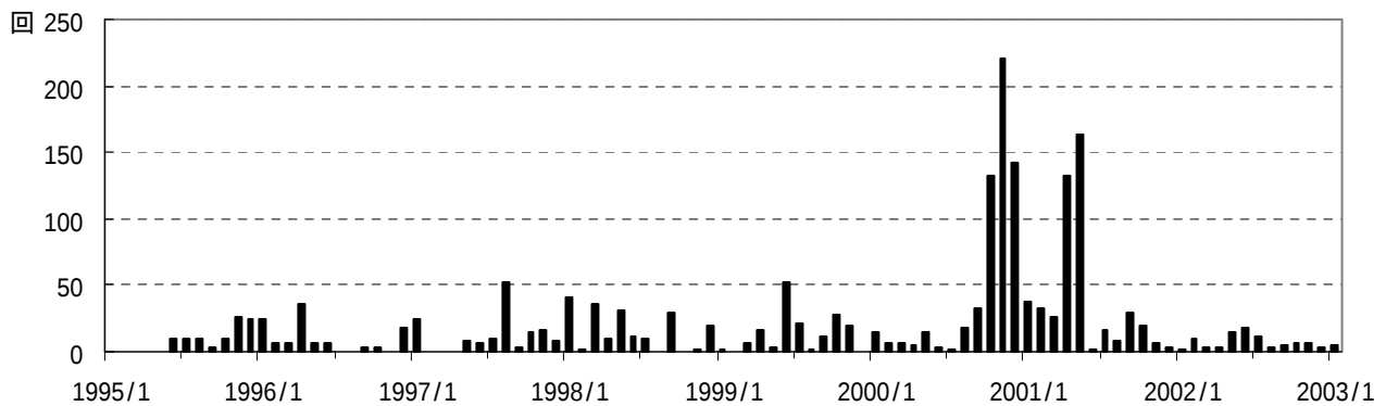
図4 富士山 低周波地震月別回数(1995年6月～2003年1月)
