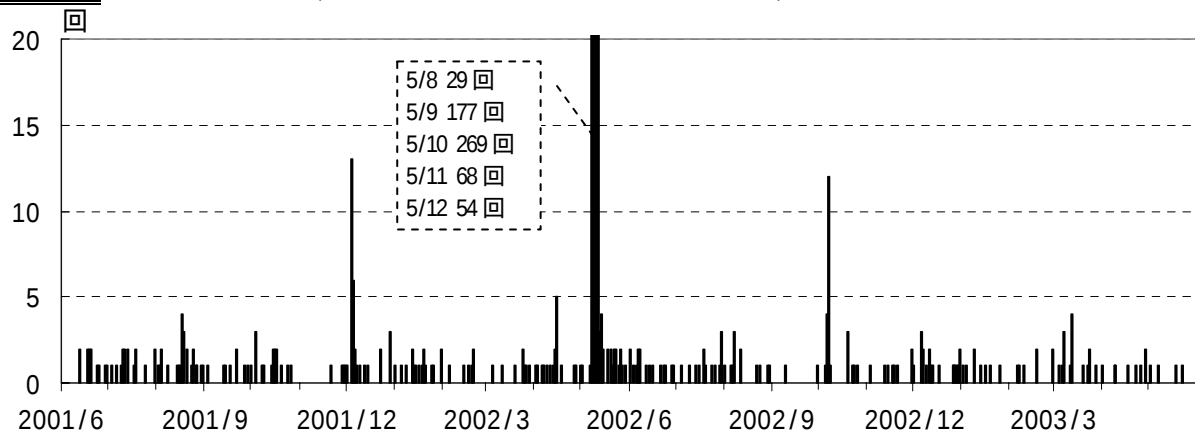
図1 伊豆東部火山群 火山性地震日別回数（2001年6月1日～2003年5月31日）
