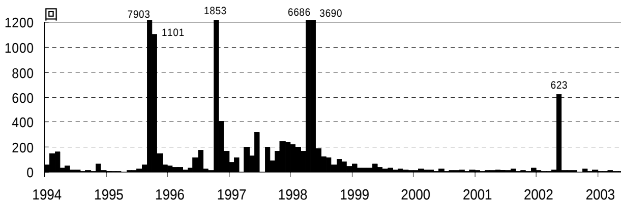
図2 伊豆東部火山群 火山性地震月別回数（1994年1月～2003年5月）
