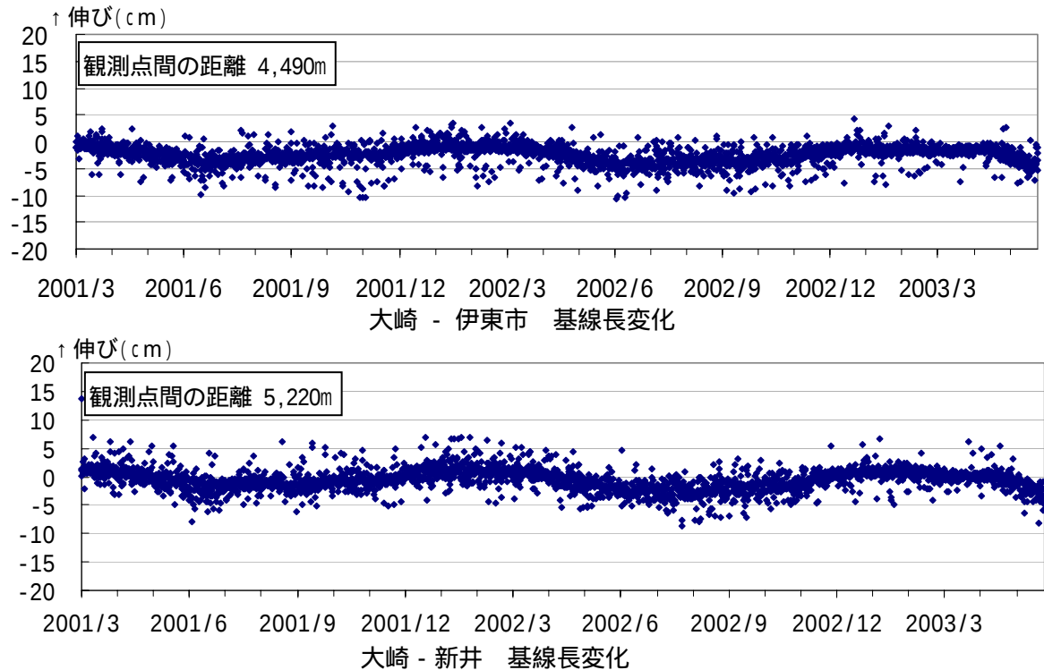
図 3 伊豆東部火山群 GPS 観測結果（2001 年 3 月 1 日～2003 年 5 月 31 日）
