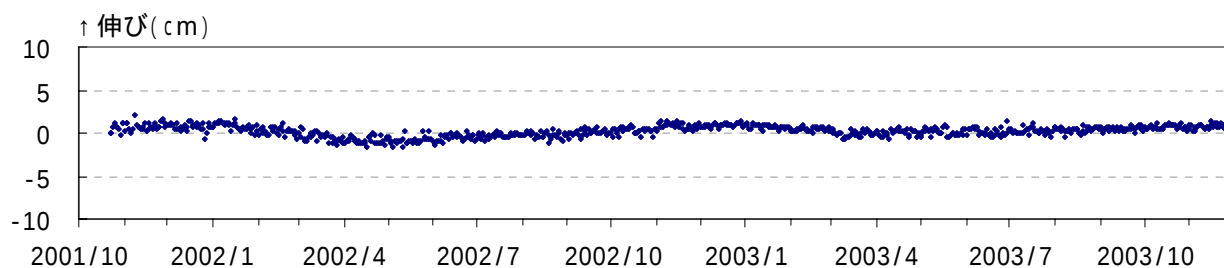
図4 御嶽山 GPS観測結果(2001年10月1日～2003年11月30日)
