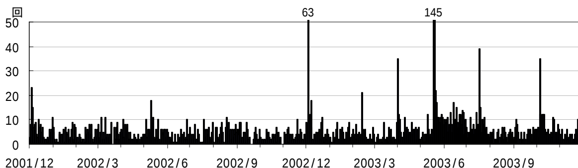
図1 御嶽山 火山性地震日別回数(2001 年 12 月 1 日～2003 年 11 月 30 日)
