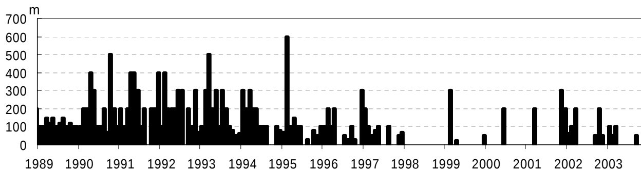
図3 御嶽山 月別最高噴煙高度 (1989年1月～2003年11月)
