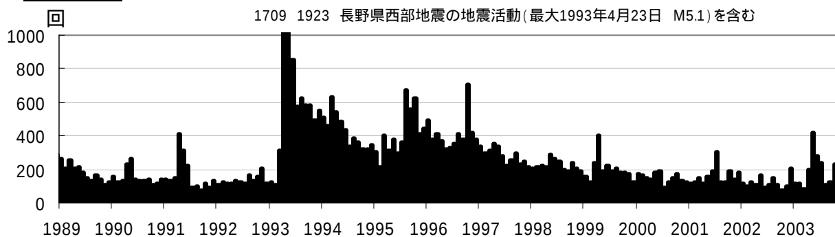
図2 御嶽山 火山性地震月別回数 (1989 年 1 月～2003 年 11 月)
