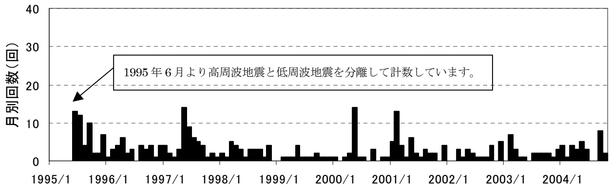
図 1 富士山 高周波地震月別回数(1995 年 6 月～2004 年 10 月)
