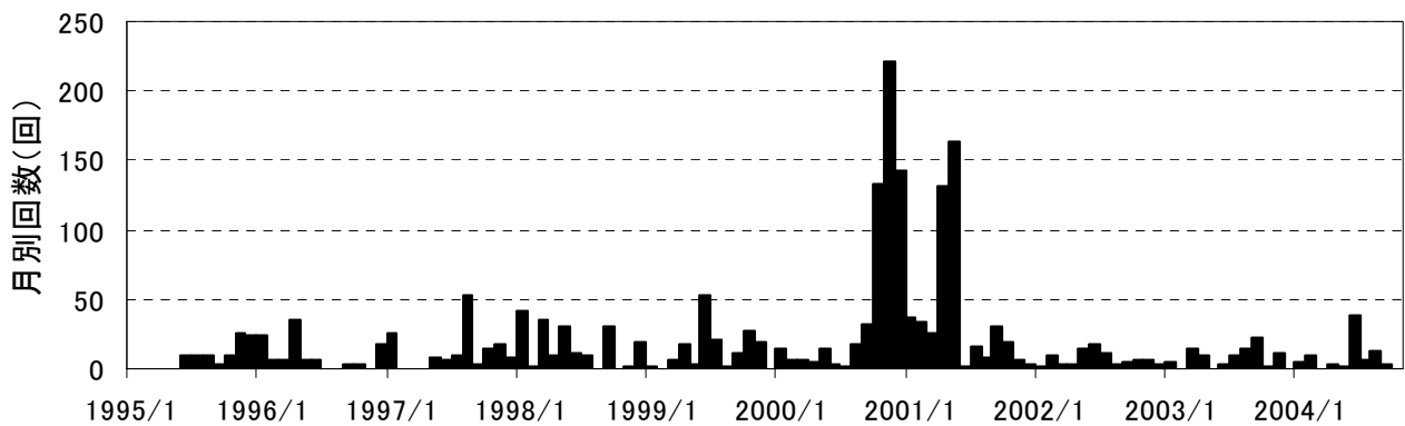
図 2 富士山 低周波地震月別回数(1995 年 6 月～2004 年 10 月)
