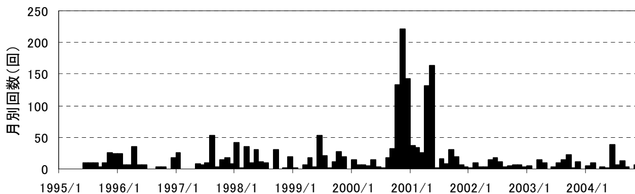
図2 富士山 低周波地震月別回数(1995年6月～2004年11月)
