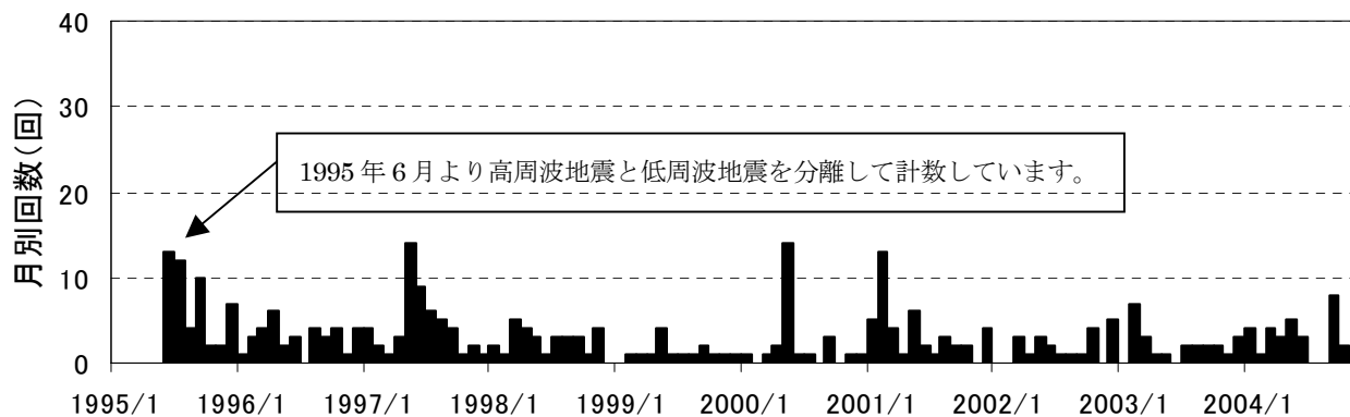
図1 富士山 高周波地震月別回数(1995年6月～2004年11月)
