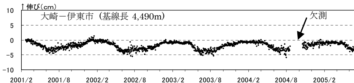
図 2 伊豆東部火山群 GPS 連続観測による基線長変化（2001 年 2 月～2005 年 6 月） その他の基線でも火山活動によるとみられる変化は観測されませんでした。
