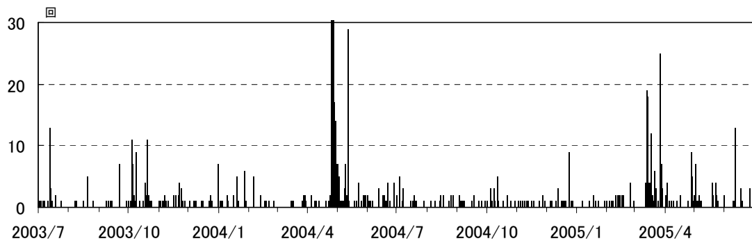
図 1 伊豆東部火山群 日別地震回数（2003 年 7 月 1 日～2005 年 6 月 30 日）
