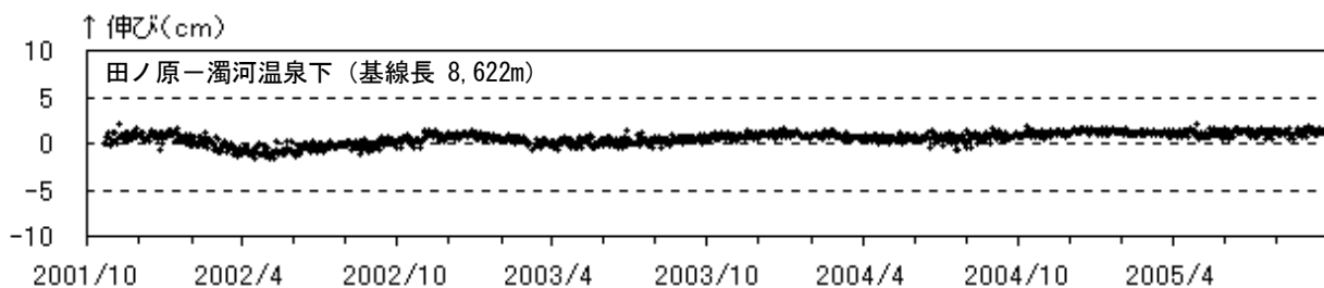
図 3 御嶽山 GPS 連続観測による基線長変化（2001 年 10 月 23 日～2005 年 9 月 30 日）
