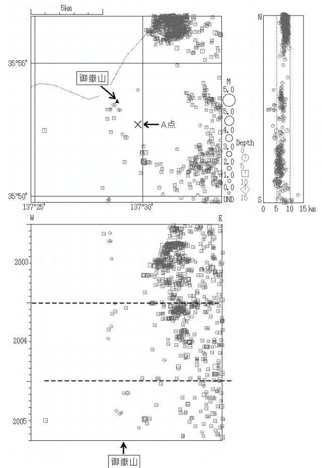
図 1 御嶽山 周辺の地震活動
