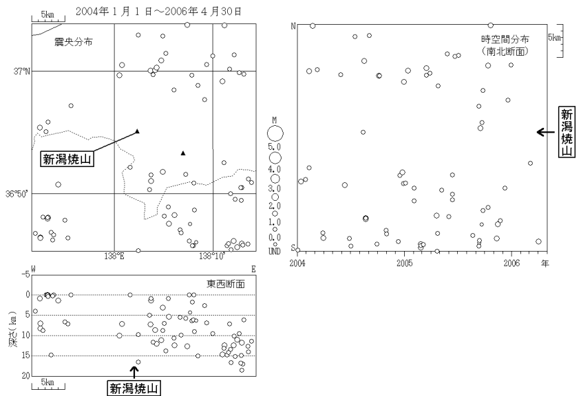
図 1 新潟焼山 広域ネットによる新潟焼山周辺の地震活動 （2004 年 1 月 1 日～2006 年 4 月 30 日）
