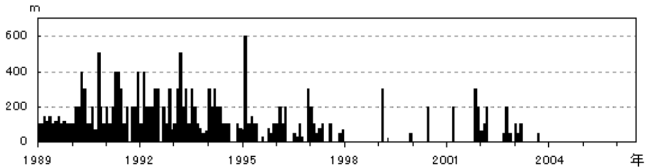
図 3 御嶽山 定時観測（09時・16時）による月別最大噴煙高度（1989年 1 月～2006 年 6 月）
