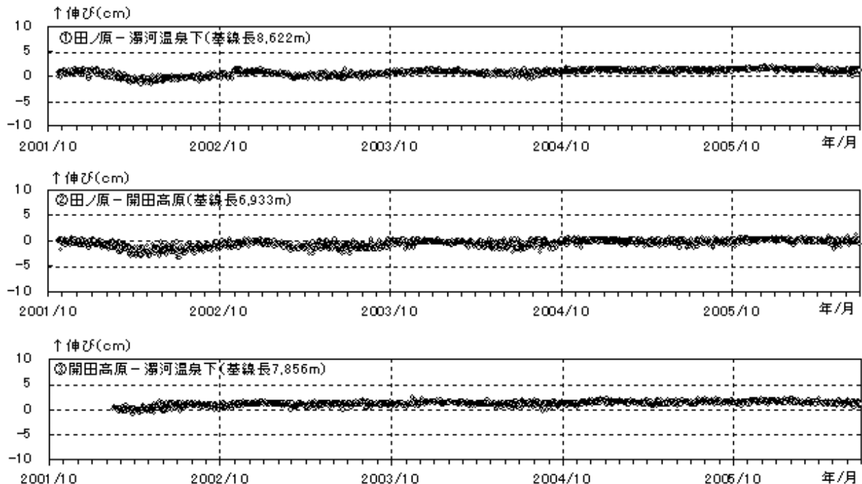
図 2 御嶽山 G P S 連続観測による基線長変化（2001 年 10 月 23 日～2006 年 6 月 30 日）
