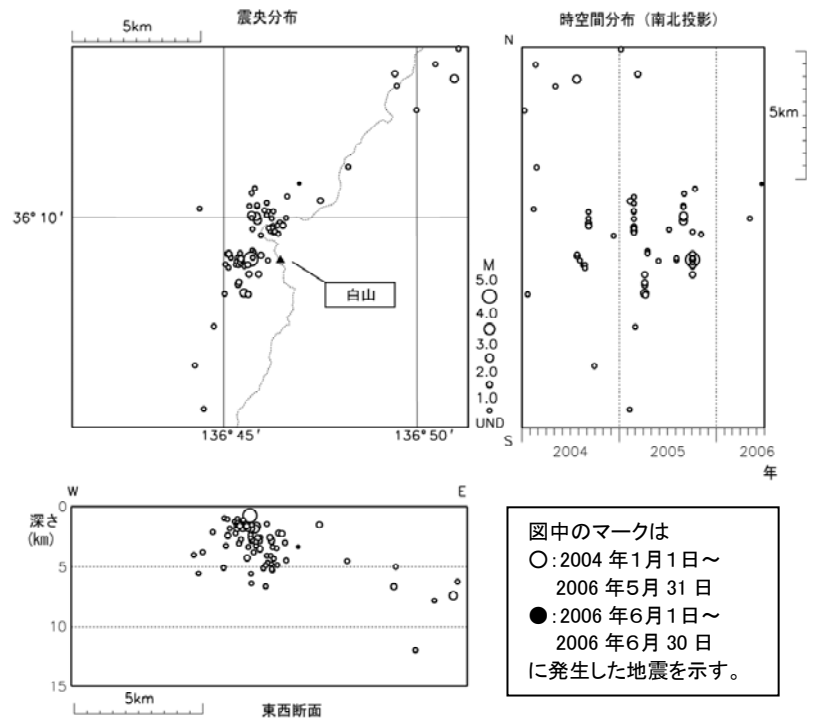
図 1 ※ 白山 山体及びその周辺の地震活動 (2004 年 1 月 1 日～2006 年 6 月 30 日)
