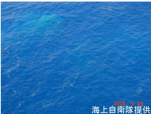
図 2 福徳岡ノ場 変色水の状況（6 月 29 日）
