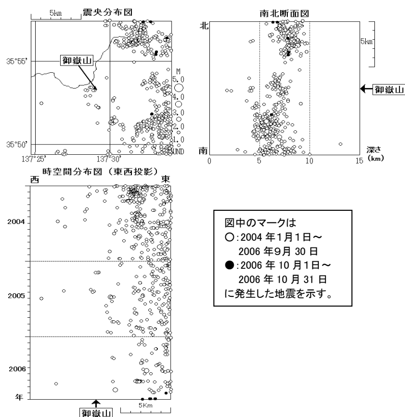
図 1 ※ 御嶽山 山体及びその周辺の地震活動 (2004 年 1 月 1 日～2006 年 10 月 31 日)
