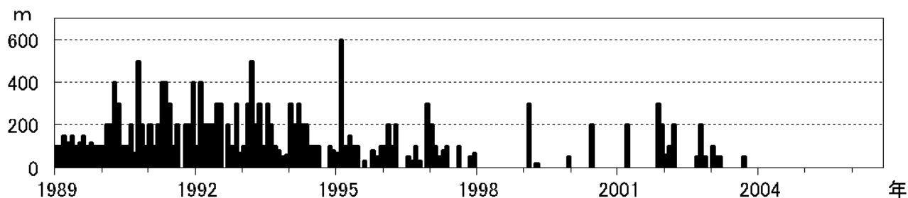
図 3 御嶽山 定時観測（09時・16時）による月別最大噴煙高度（1989年 1 月～2006年10月）
