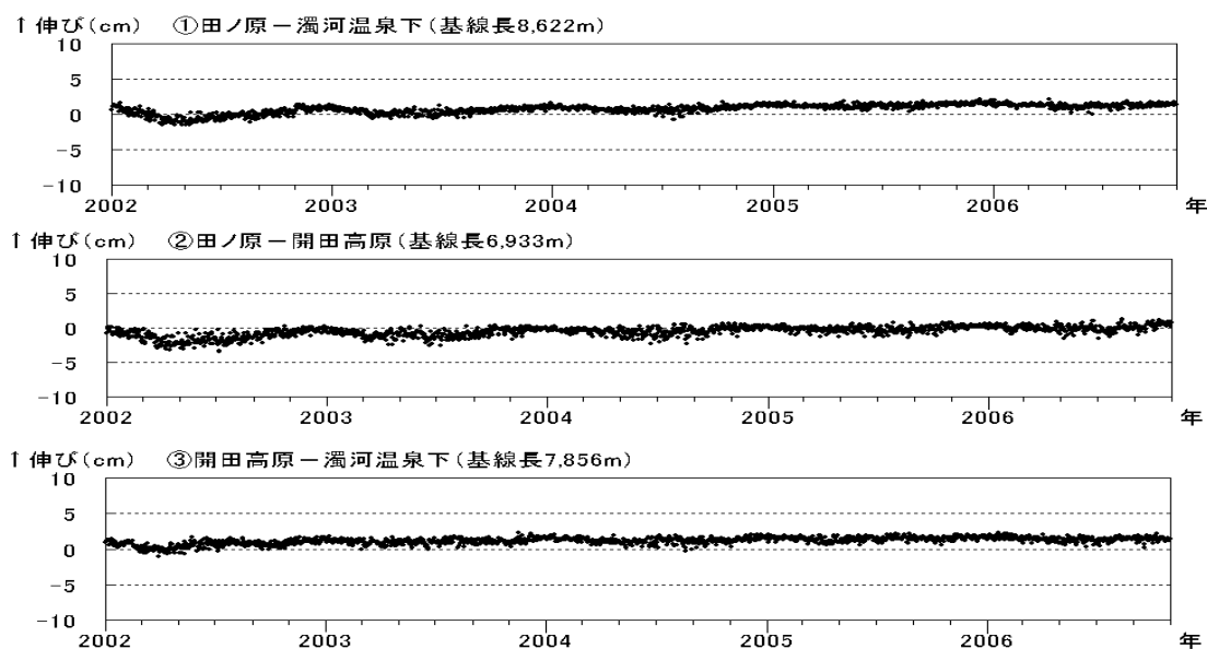
図 2 御嶽山 G P S 連続観測による基線長変化（2002 年 1 月 1 日～2006 年 10 月 31 日）
